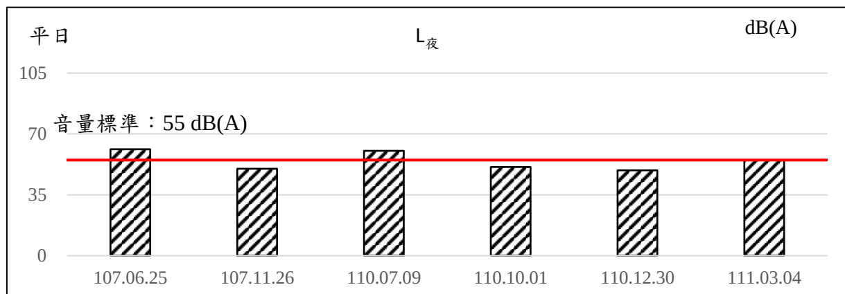
圖2.2-6、歷次鐵道之鄉酒莊測站噪音監測結果變化情形
