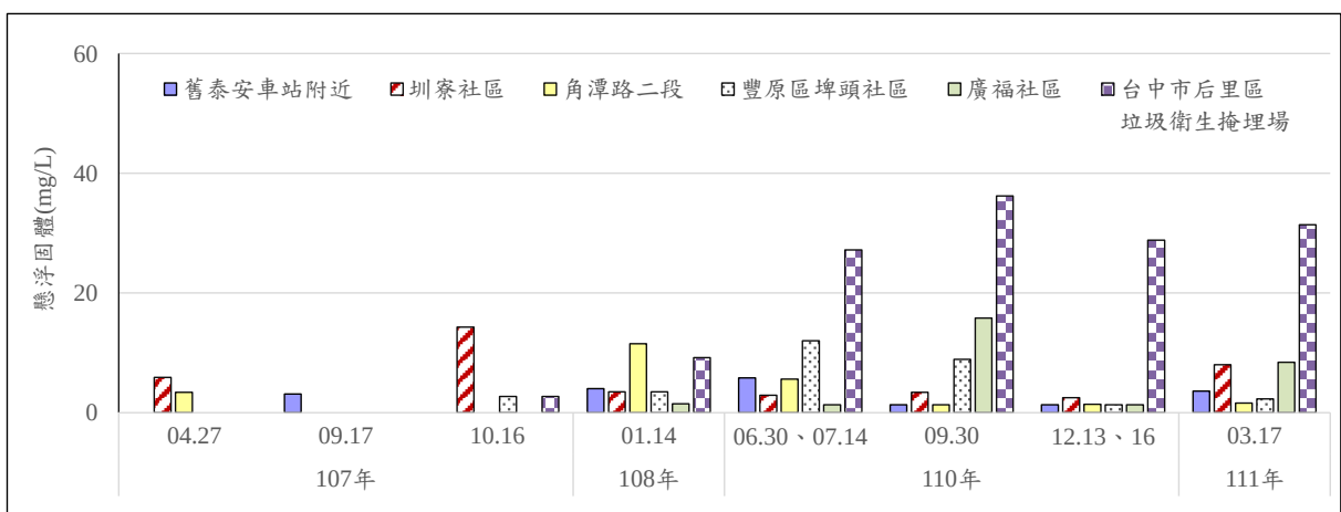
圖2.5-2、歷次地下水監測結果變化情形
