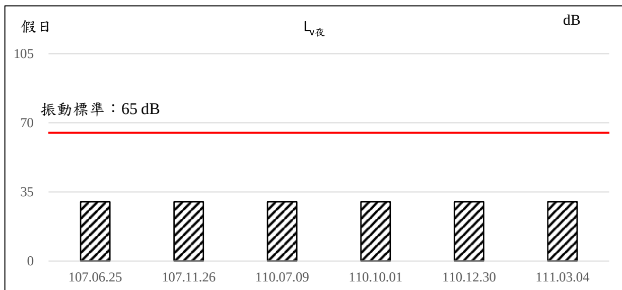
圖2.2-13、歷次豐原區埤頭社區測站振動監測結果變化情形(續1)
