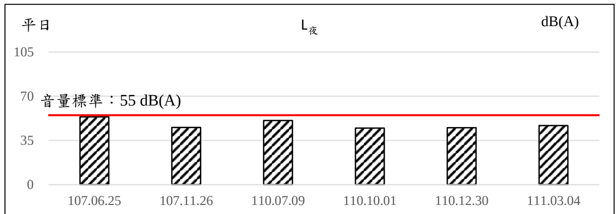
圖2.2-5、歷次廣福社區測站噪音監測結果變化情形
