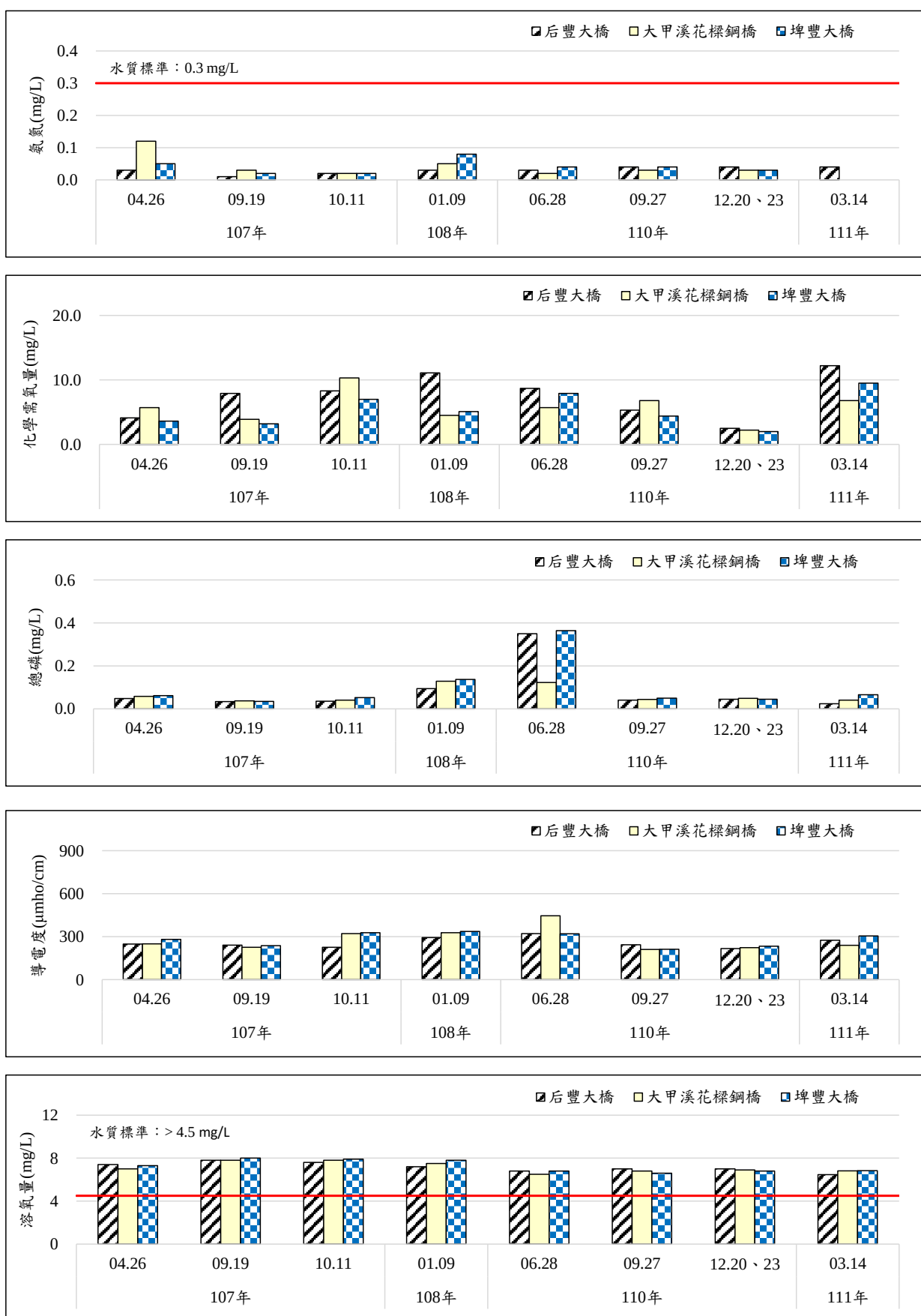
圖2.3-3、歷次河川水質監測結果變化情形(大甲溪測站_丙類水體)(續)
