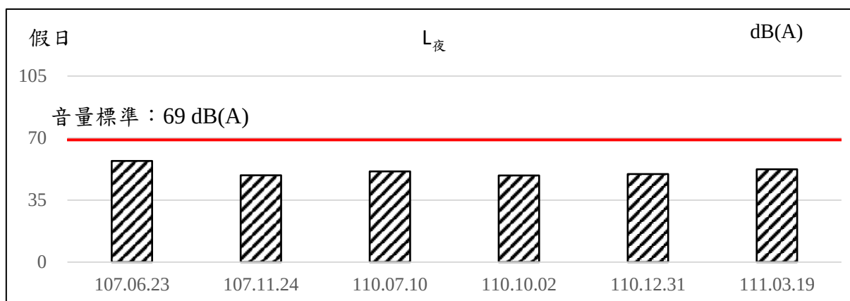
圖2.2-3、歷次舊泰安車站附近測站噪音監測結果變化情形(續1)
