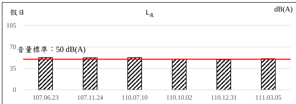
圖2.2-7、歷次豐原區埤頭社區測站噪音監測結果變化情形(續1)
