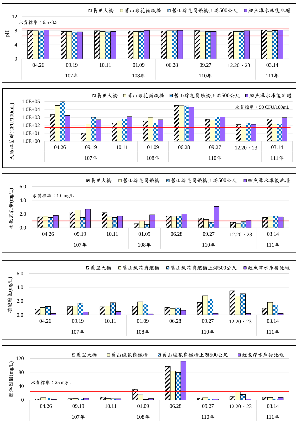
圖2.3-2、歷次河川水質監測結果變化情形(大安溪測站)
