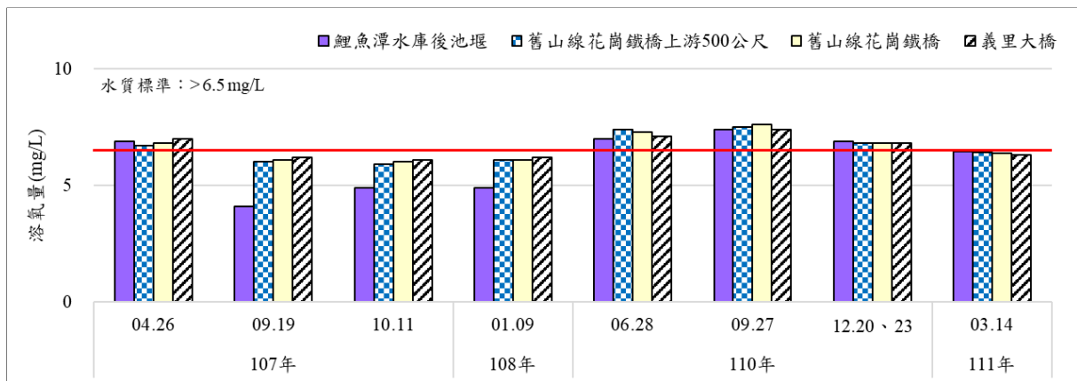
圖 3.1.2-3、歷年大安溪測站河川水質監測結果趨勢圖
