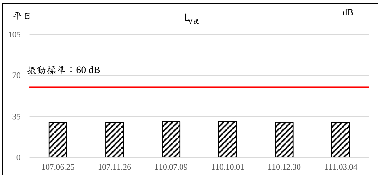
圖2.2-8、歷次鯉魚潭水庫管理中心測站振動監測結果變化情形
