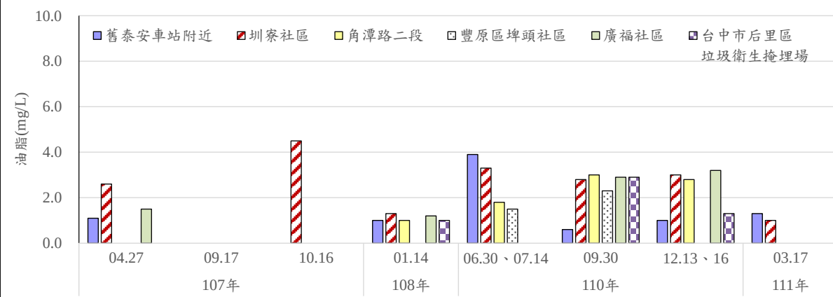
圖2.5-2、歷次地下水監測結果變化情形(續1)
