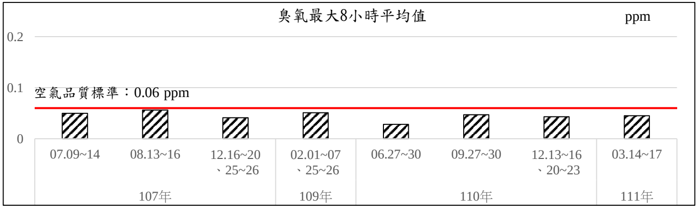
圖2.1-3、歷次舊泰安車站附近測站空氣品質監測結果變化情形(續2)
