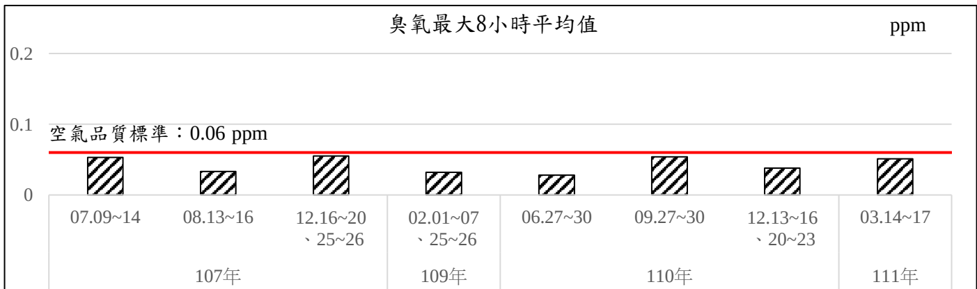
圖2.1-5、歷次廣福社區測站空氣品質監測結果變化情形(續2)
