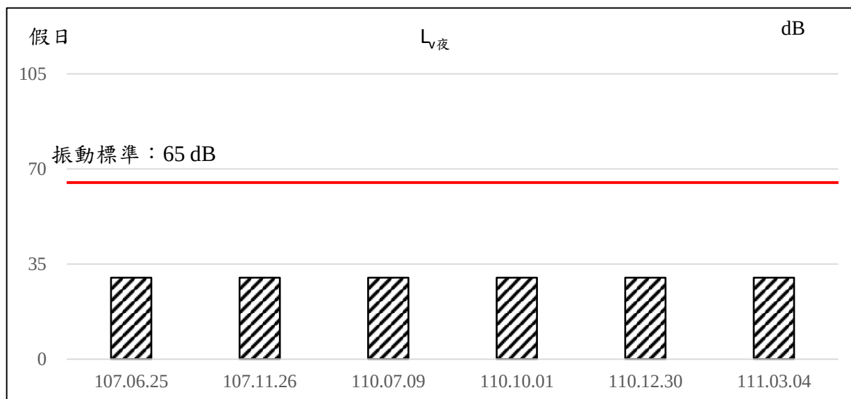
圖2.2-12、歷次鐵道之鄉酒莊測站振動監測結果變化情形(續1)
