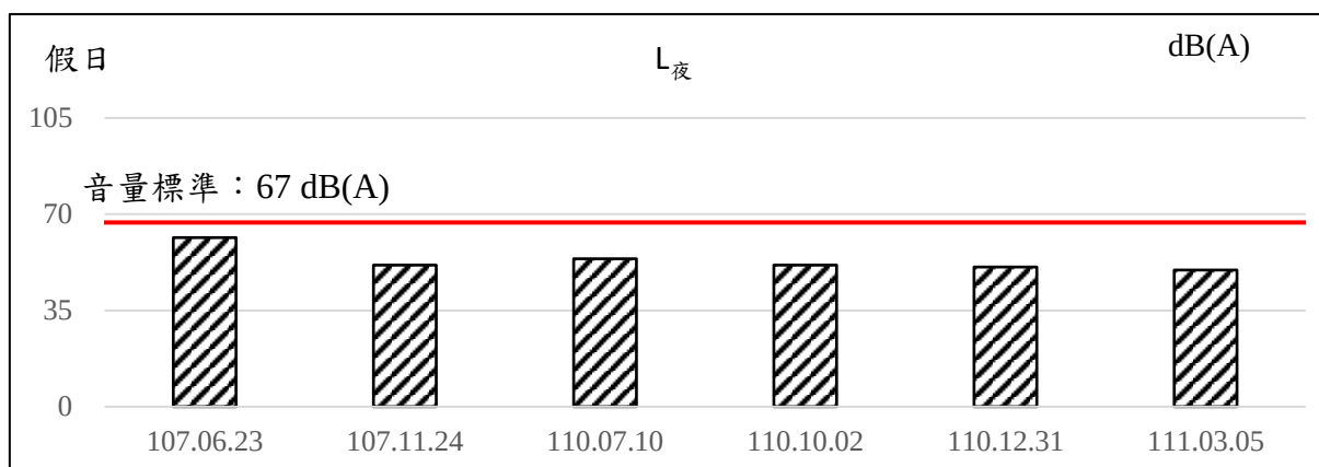
圖2.2-2、歷次鯉魚潭水庫管理中心測站噪音監測結果變化情形(續1)
