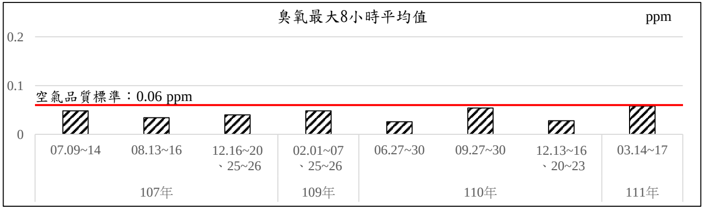
圖2.1-7、歷次豐原區埤頭社區測站空氣品質監測結果變化情形(續2)
