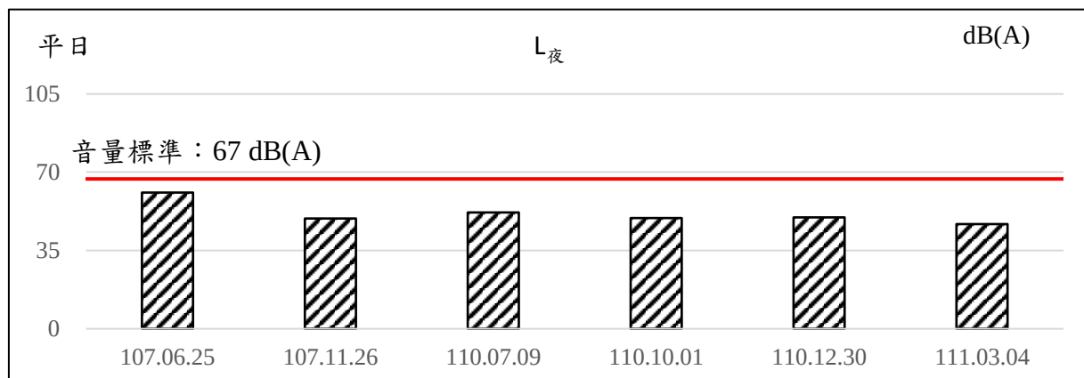
圖2.2-2、歷次鯉魚潭水庫管理中心測站噪音監測結果變化情形
