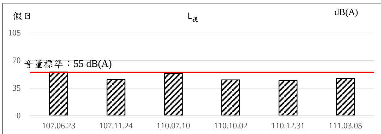
圖2.2-5、歷次廣福社區測站噪音監測結果變化情形(續1)
