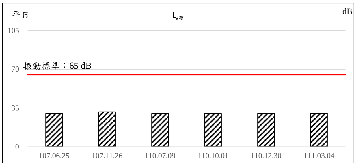
圖2.2-10、歷次圳寮社區測站振動監測結果變化情形
