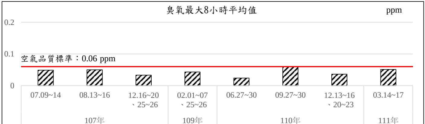
圖2.1-6、歷次鐵道之鄉酒莊測站空氣品質監測結果變化情形(續2)
