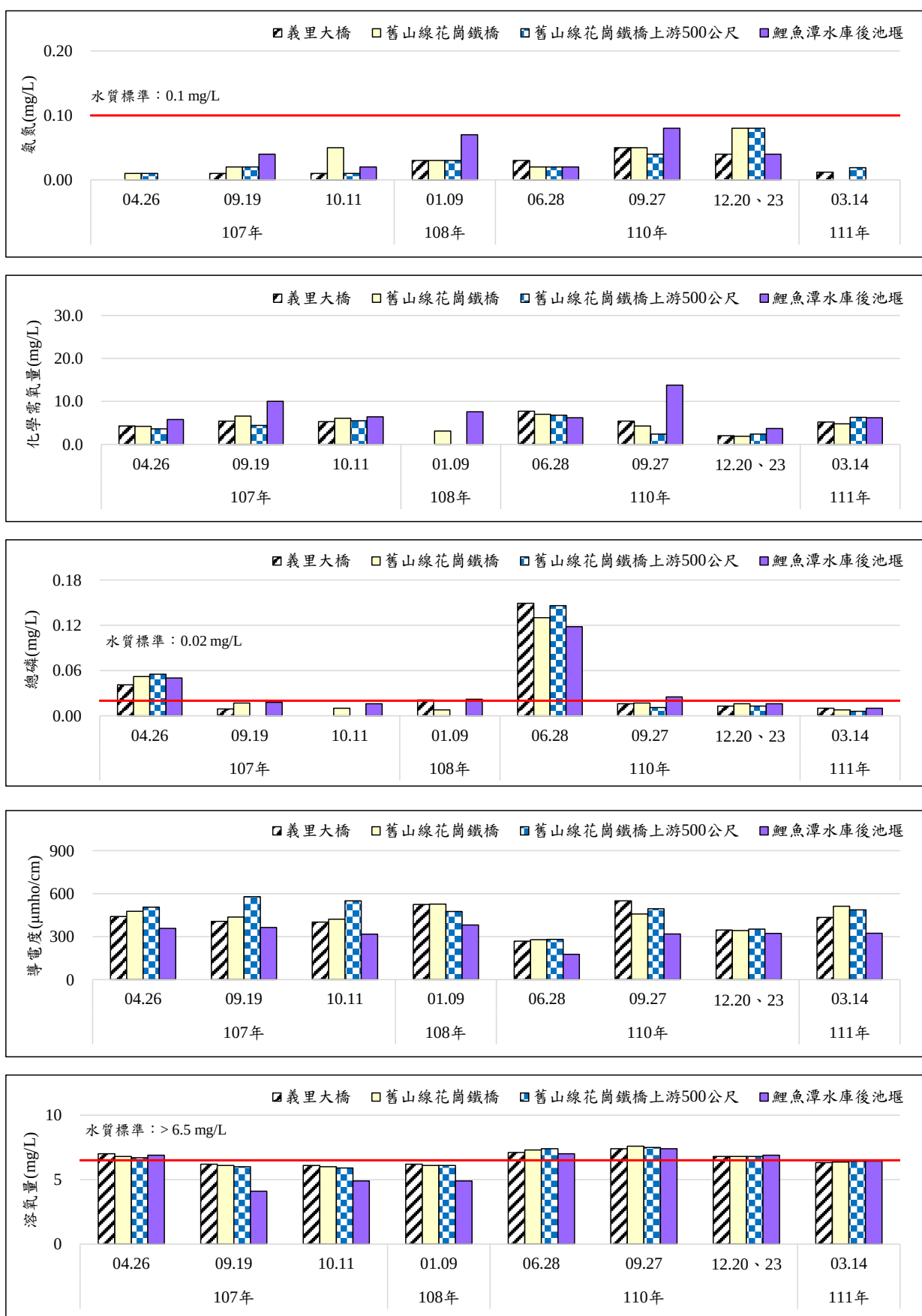
圖2.3-2、歷次河川水質監測結果變化情形(大安溪測站)(續)
