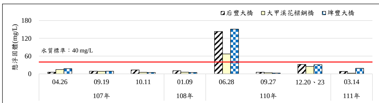
圖2.3-3、歷次河川水質監測結果變化情形(大甲溪測站_丙類水體)
