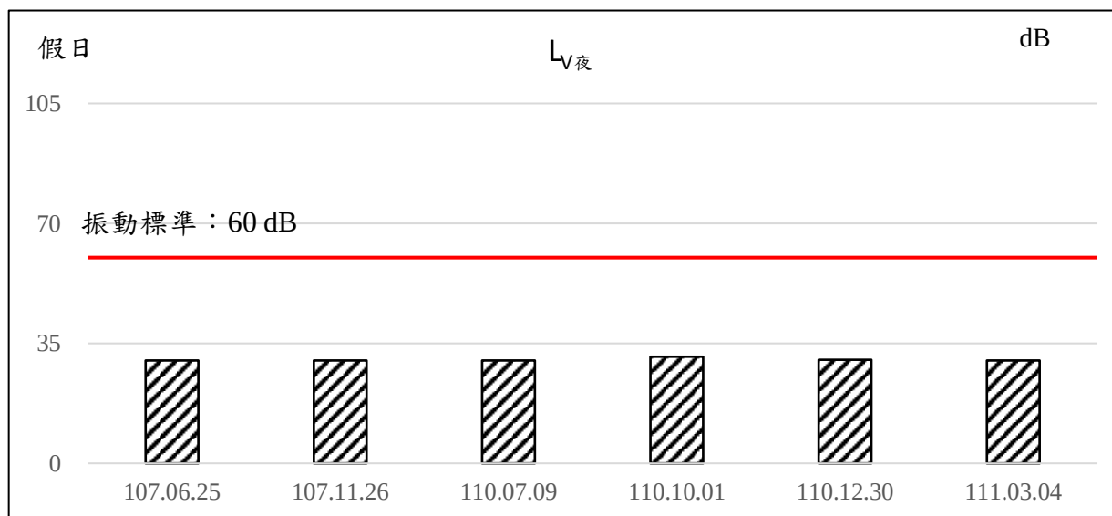
圖2.2-8、歷次鯉魚潭水庫管理中心測站振動監測結果變化情形(續1)
