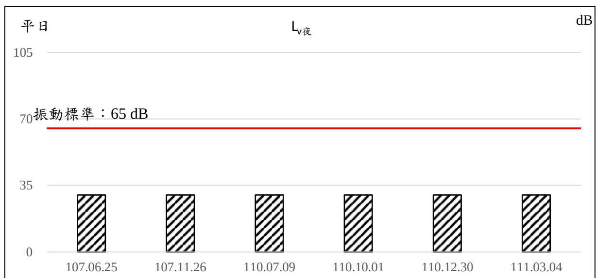
圖2.2-13、歷次豐原區埤頭社區測站振動監測結果變化情形
