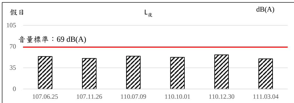
圖2.2-4、歷次圳寮社區測站噪音監測結果變化情形(續1)
