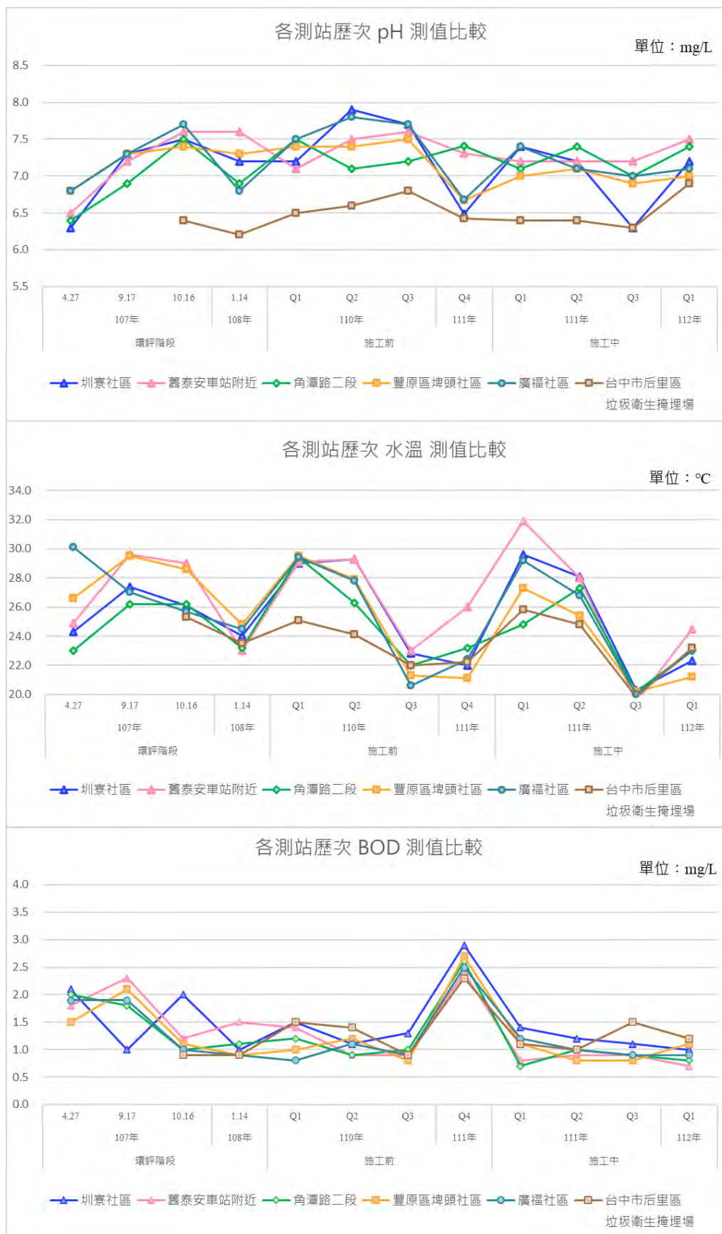
圖3.1.1-23 歷次地下水監測結果變化情形
