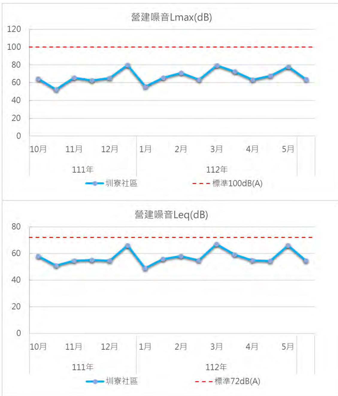
圖3.1.1-17 圳寮社區測站歷次營建噪音監測結果變化情形
