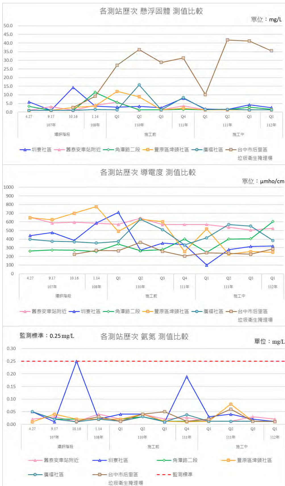
圖3.1.1-23 歷次地下水監測結果變化情形(續1)
