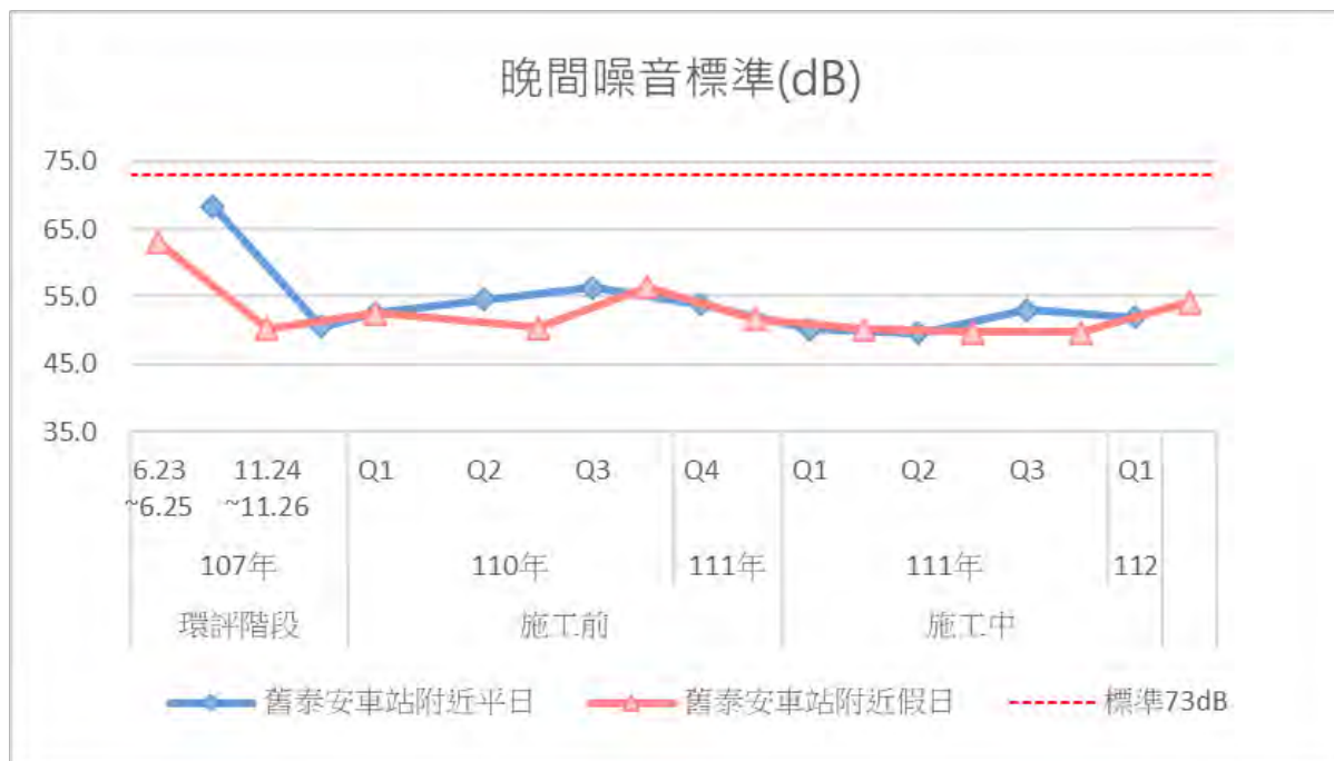
圖3.1.1-3 歷次舊泰安車站附近測站噪音監測結果變化情形
