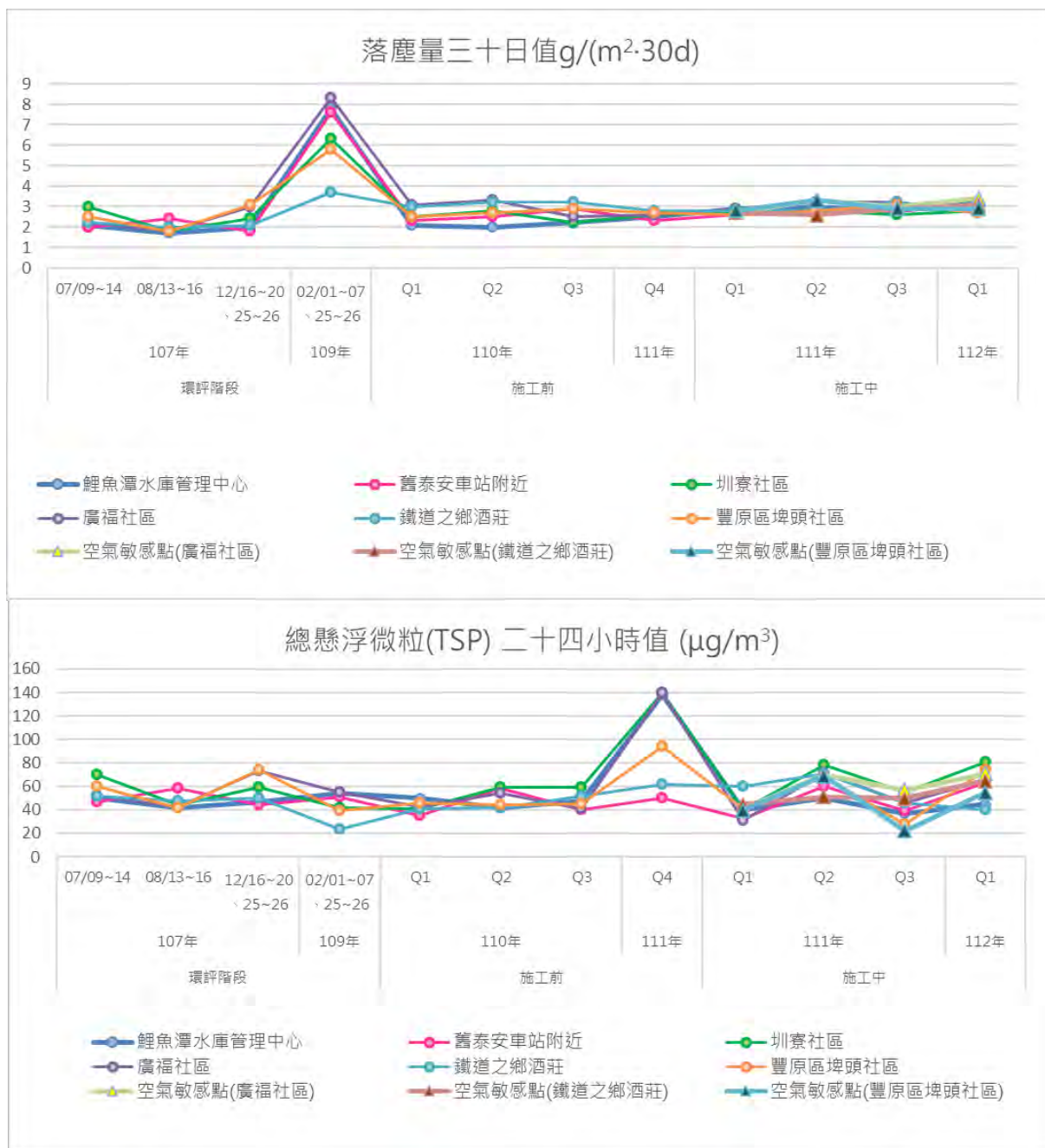
圖3.1.1-1 歷次空氣品質監測結果變化情形
