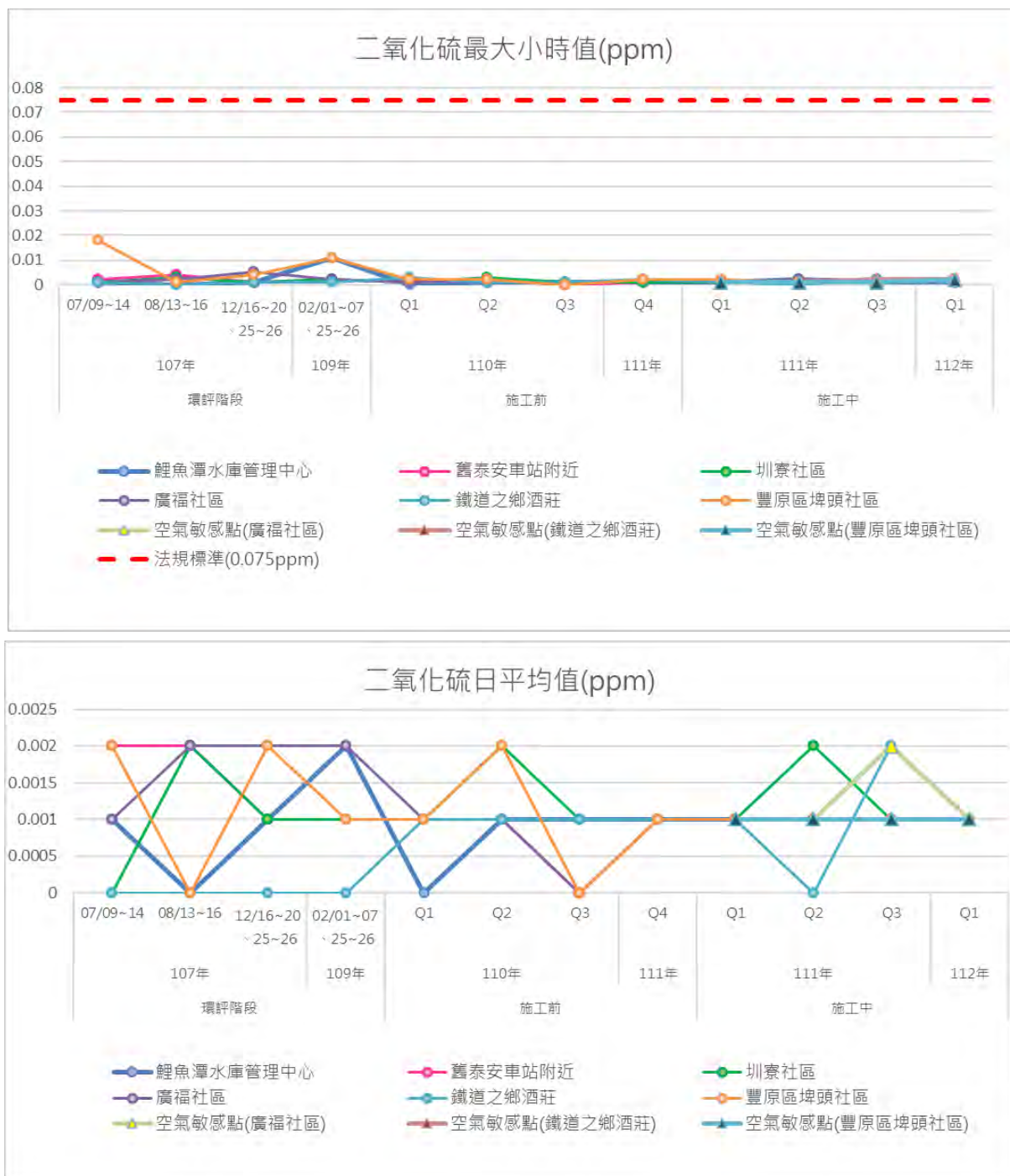
圖3.1.1-1 歷次空氣品質監測結果變化情形(續4)
