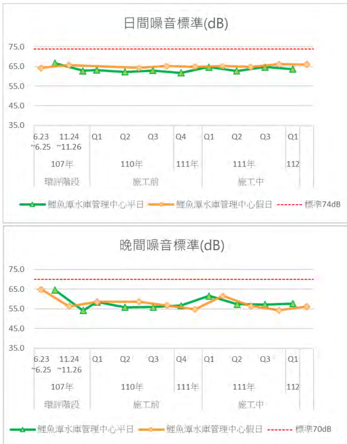
圖3.1.1-2 歷次鯉魚潭水庫管理中心測站噪音監測結果變化情形
