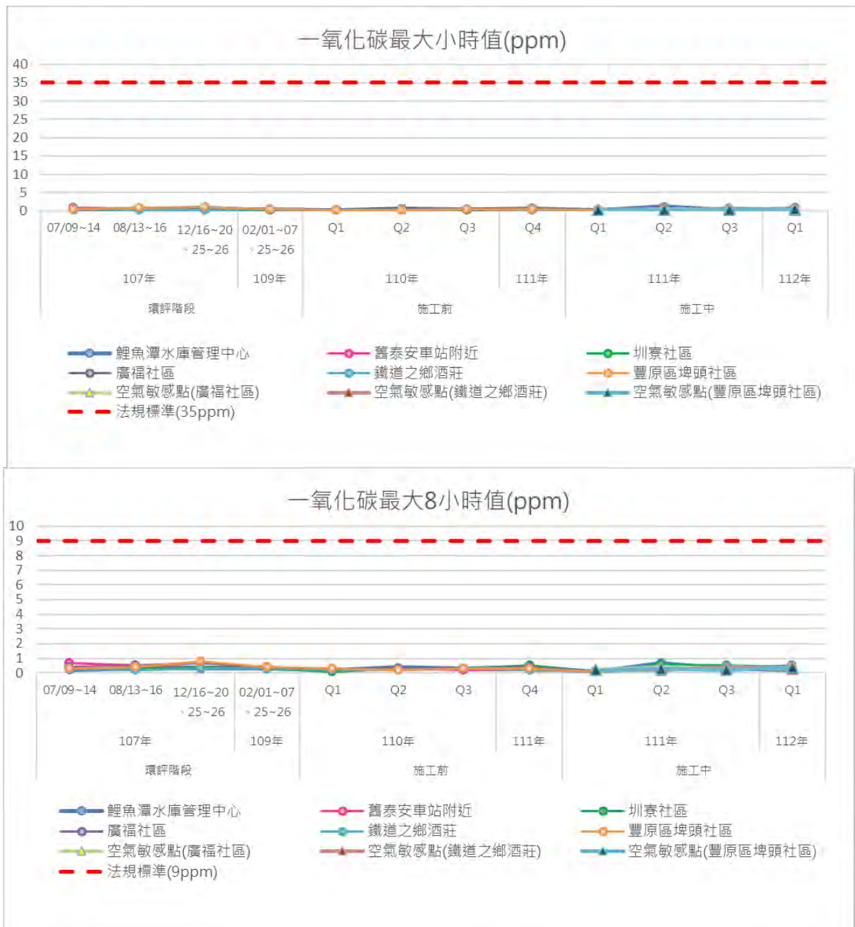
圖3.1.1-1 歷次空氣品質監測結果變化情形(續7)
