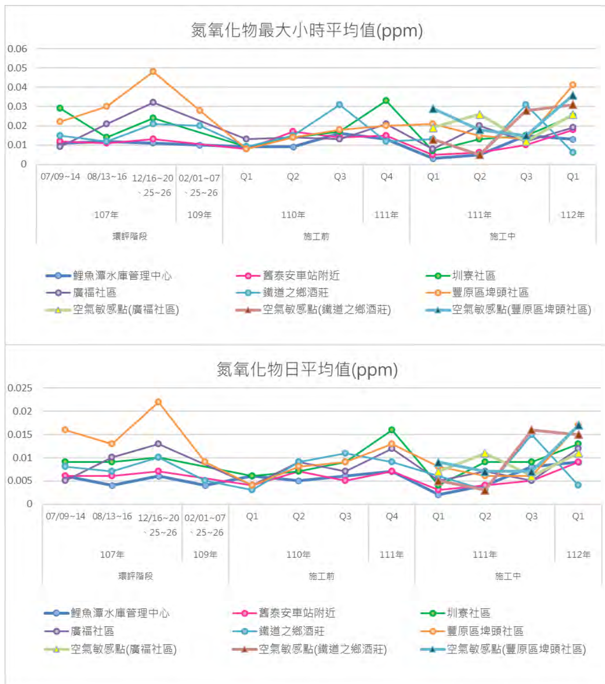
圖3.1.1-1 歷次空氣品質監測結果變化情形(續6)
