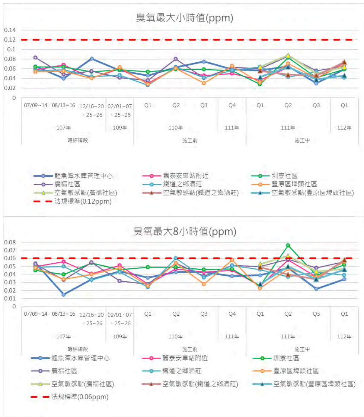
圖3.1.1-1 歷次空氣品質監測結果變化情形(續2)
