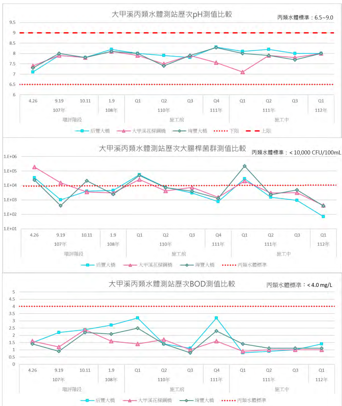
圖3.1.1-21 歷次河川水質監測結果變化情形(大甲溪丙類水體測站)
