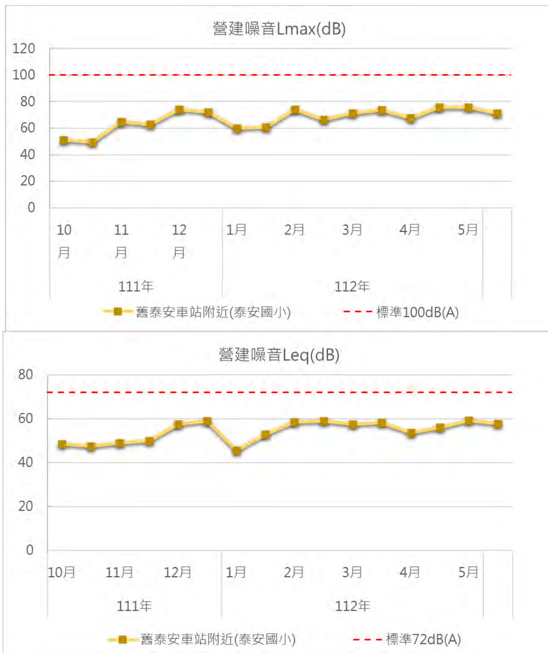
圖3.1.1-16 舊泰安車站附近(泰安國小)測站歷次營建噪音監測結果變化情形
