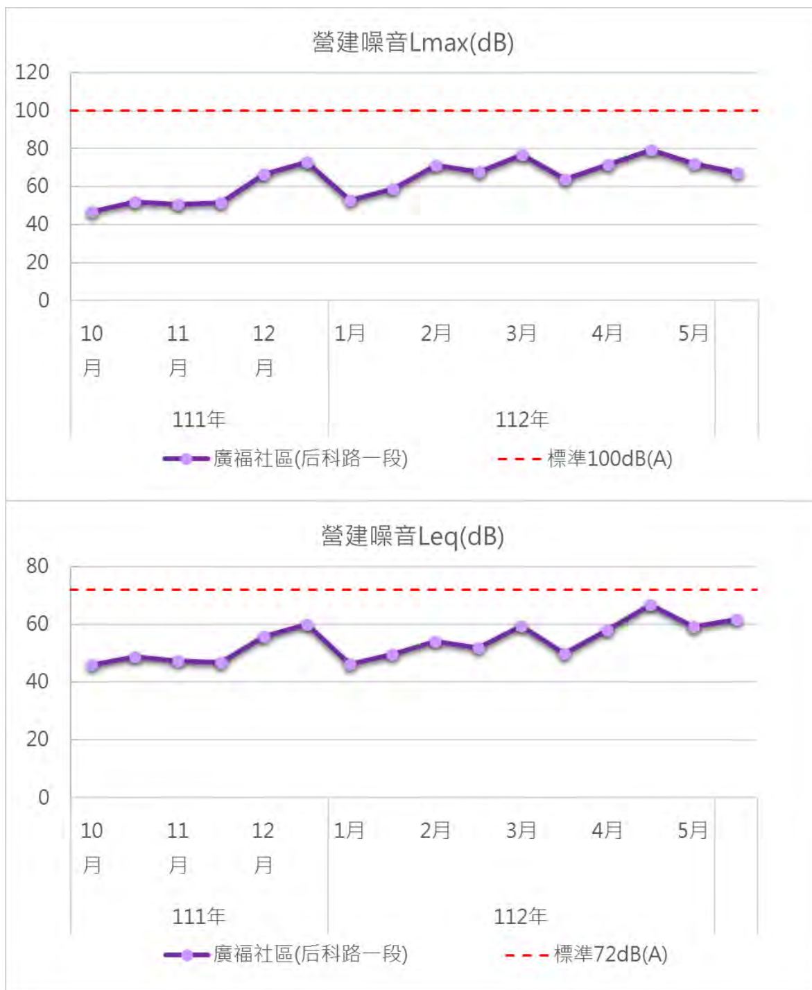
圖3.1.1-18 廣福社區測站歷次營建噪音監測結果變化情形
