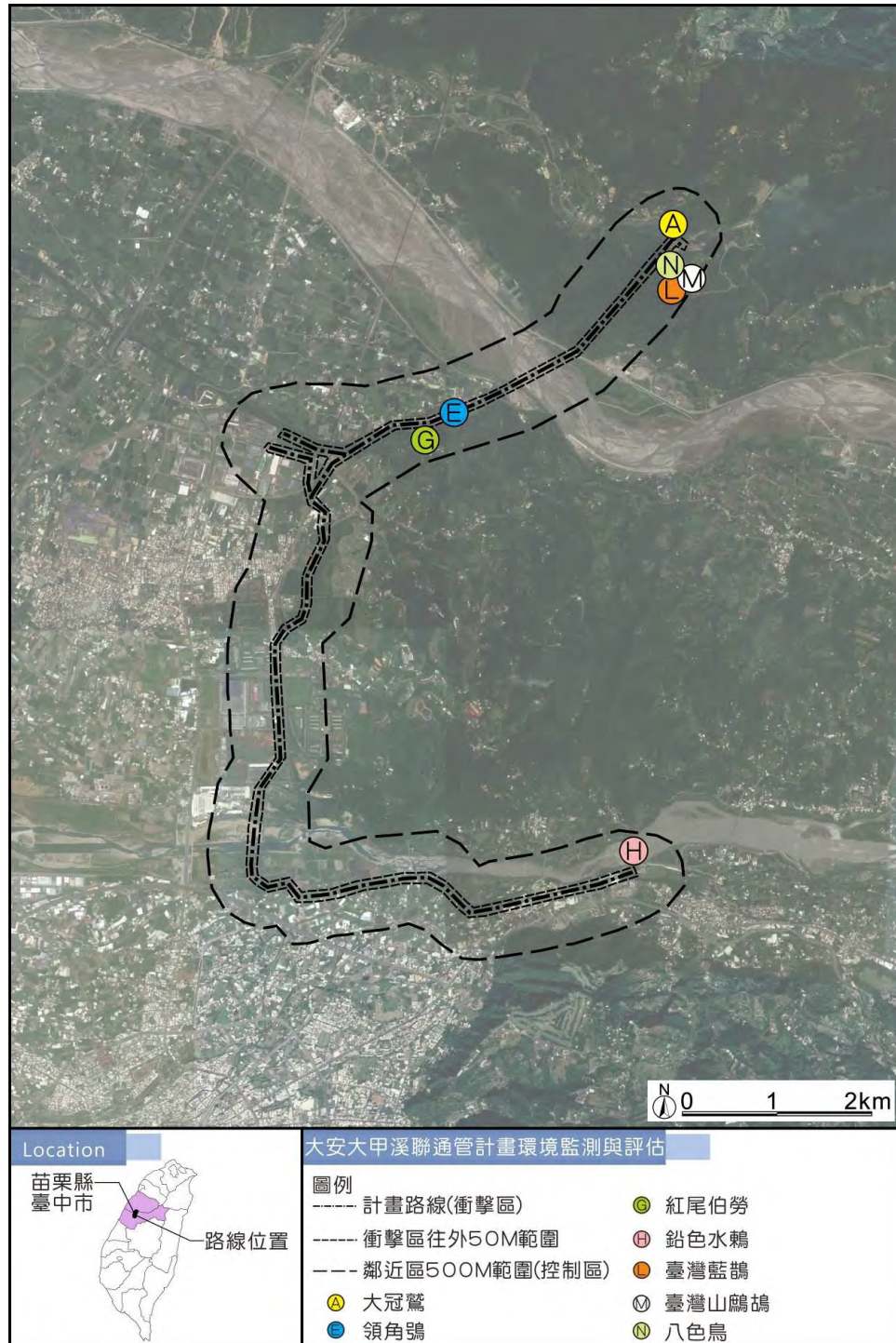
圖2.8.1-1 本季鳥類保育類動物分布圖
