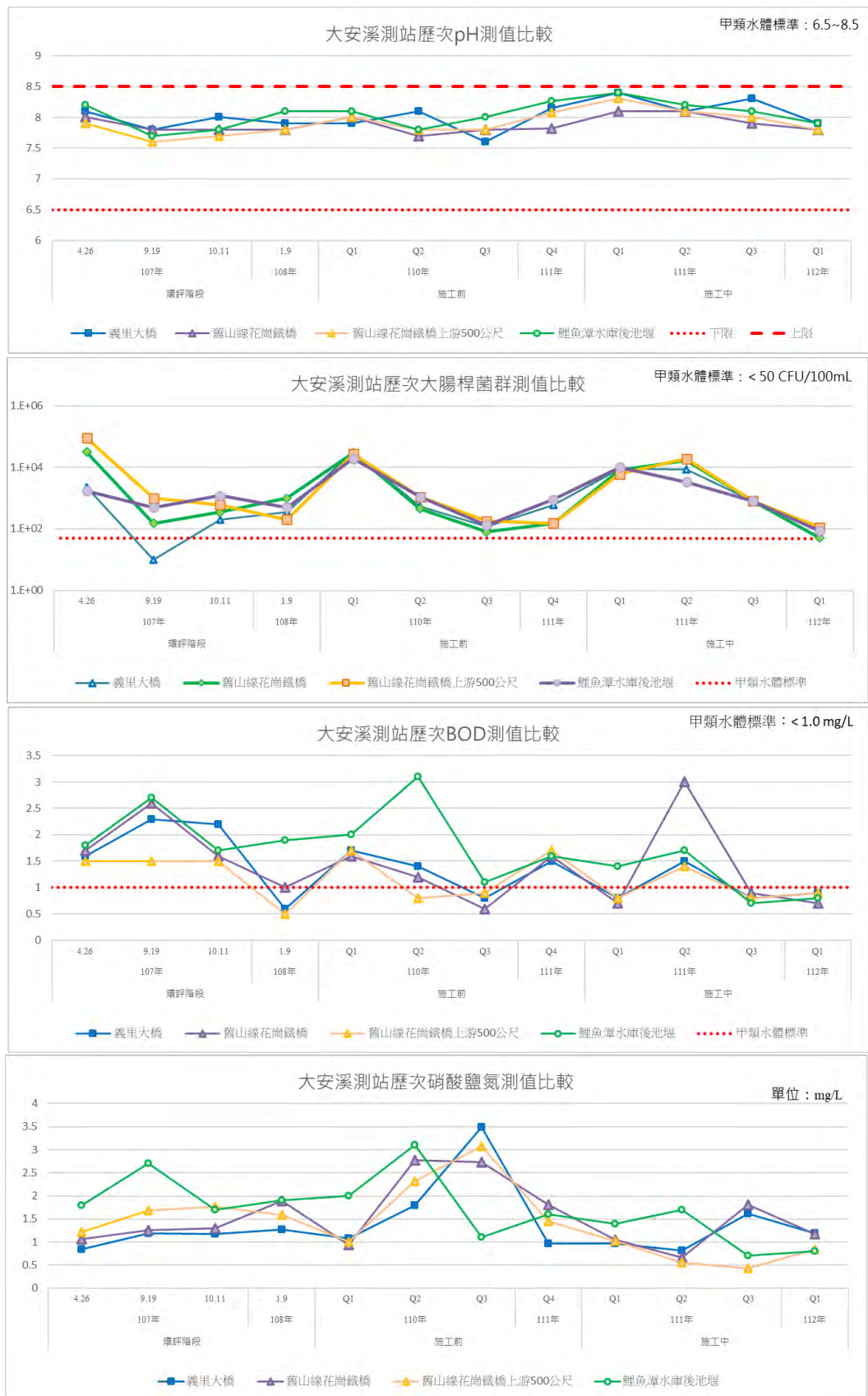
圖 3.1.1-20 歷次河川水質監測結果變化情形(大安溪測站)
