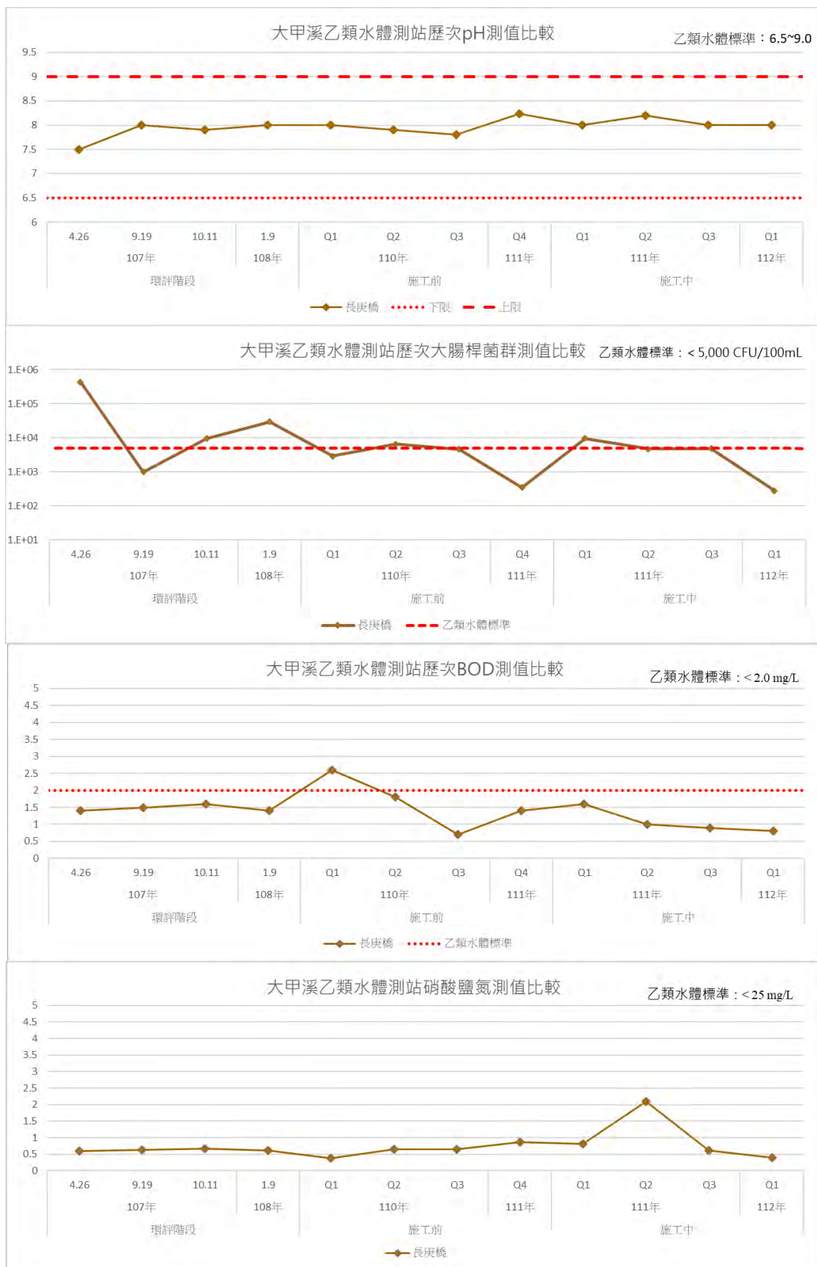
圖3.1.1-22 歷次河川水質監測結果變化情形(大甲溪乙類水體測站)
