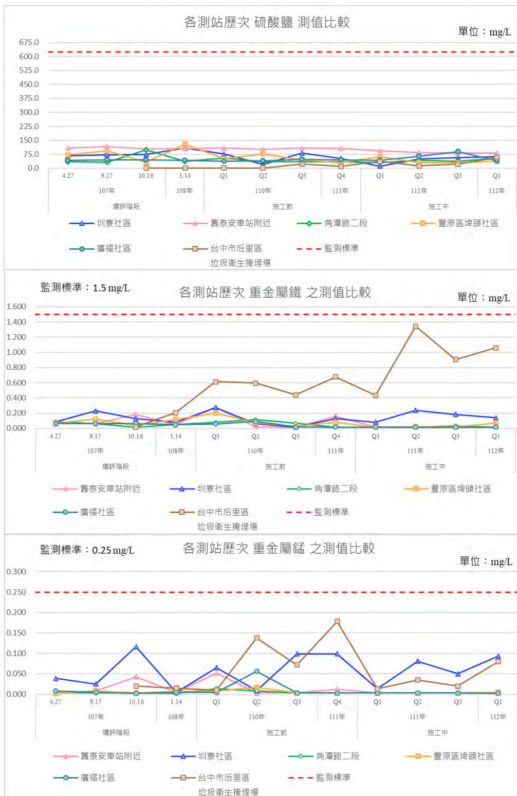
圖3.1.1-23 歷次地下水監測結果變化情形(續3)
