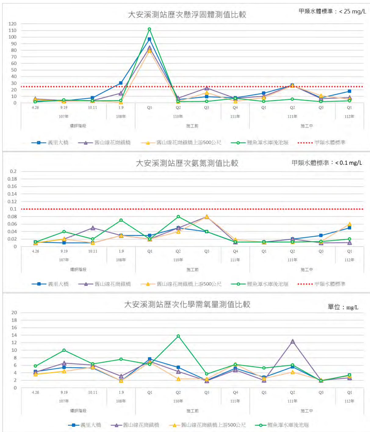
圖3.1.1-20 歷次河川水質監測結果變化情形(大安溪測站)(續1)
