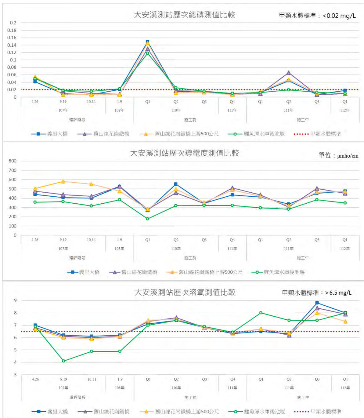
圖3.1.1-20 歷次河川水質監測結果變化情形(大安溪測站)(續2)
