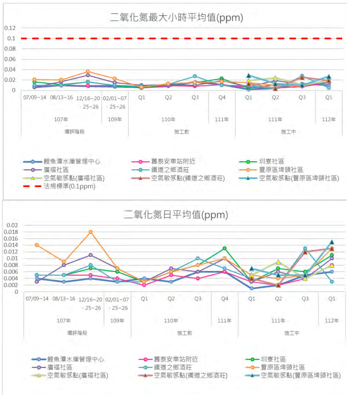
圖3.1.1-1 歷次空氣品質監測結果變化情形(續5)
