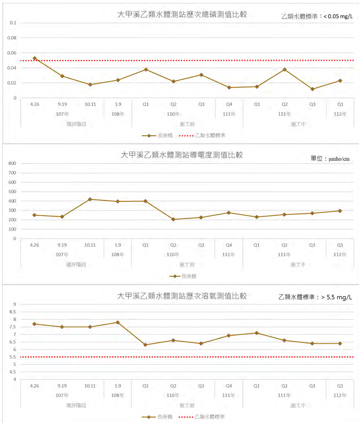
圖3.1.1-22 歷次河川水質監測結果變化情形(大甲溪乙類水體測站)(續2)
