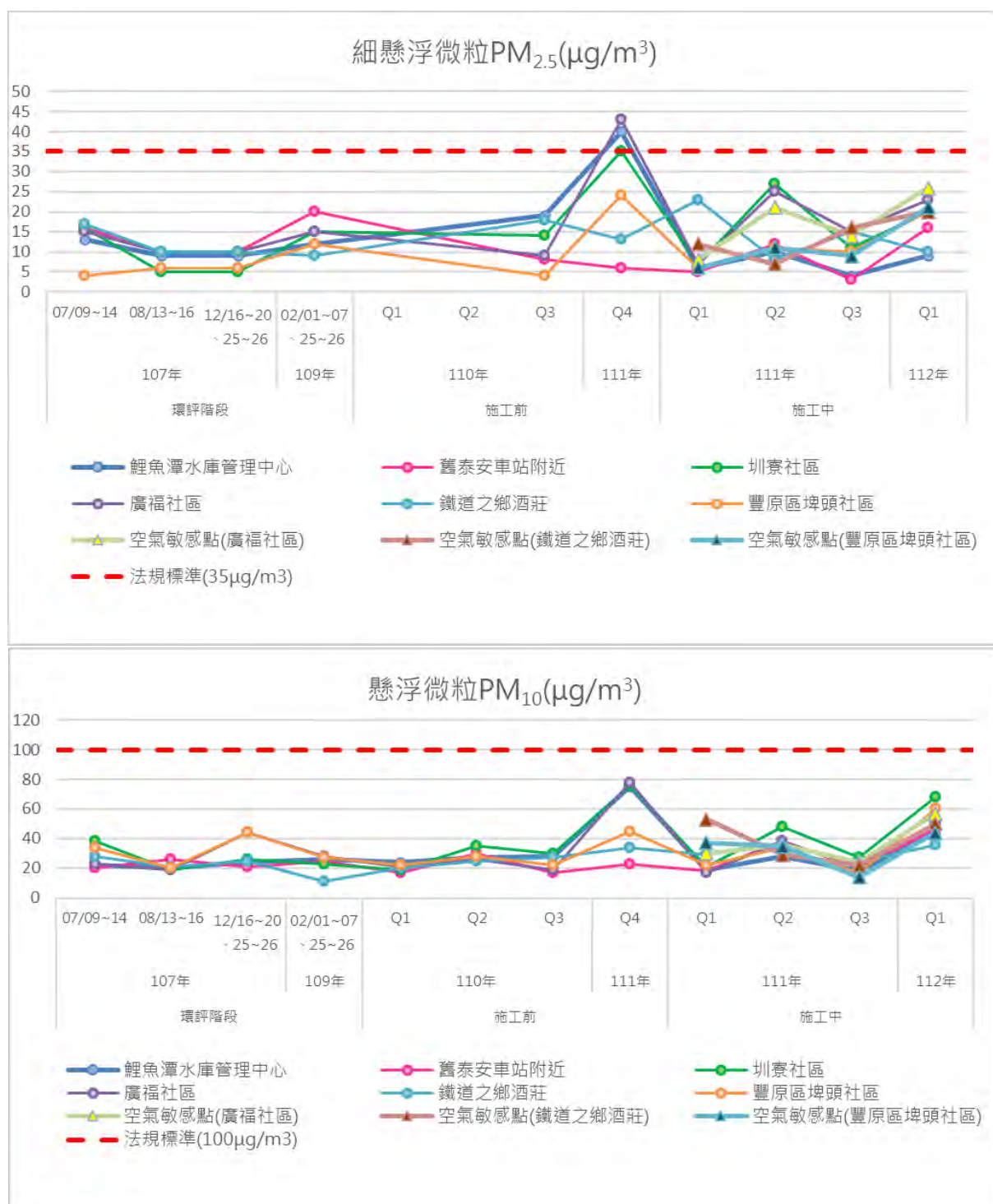
圖3.1.1-1 歷次空氣品質監測結果變化情形(續3)
