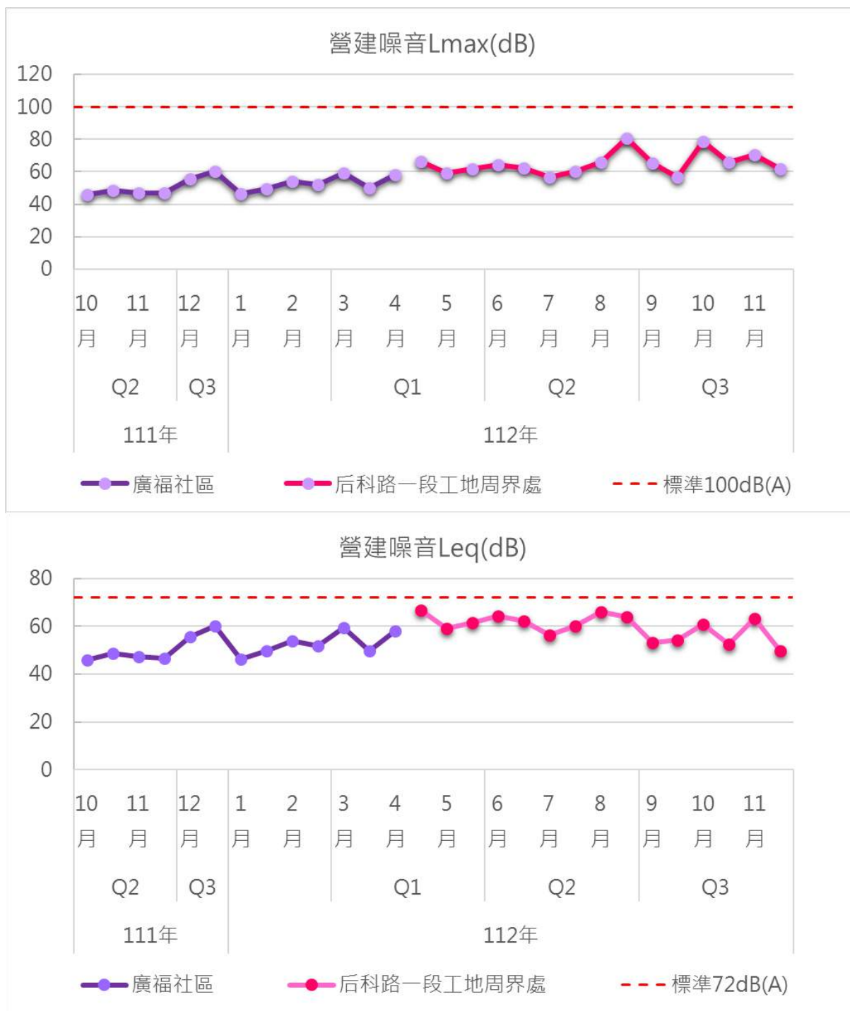
圖3.1.1-18 廣福社區測站及后科路一段工地周界處測站歷次營建噪音監測結果變化情形
