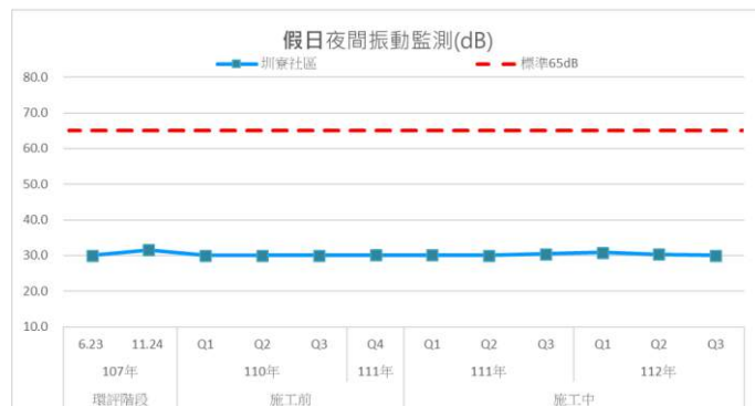
圖3.1.1-10 歷次圳寮社區測站振動監測結果變化情形
