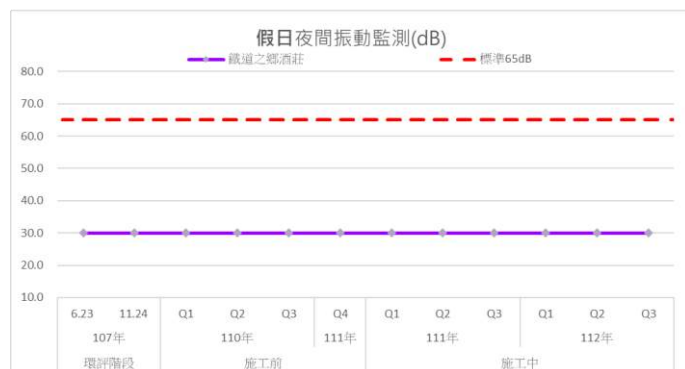
圖3.1.1-12 歷次鐵道之鄉酒莊測站振動監測結果變化情形
