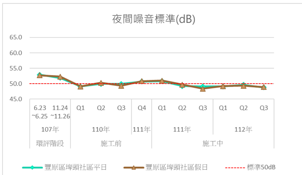
圖3.1.1-7 歷次豐原區埤頭社區測站噪音監測結果變化情形
