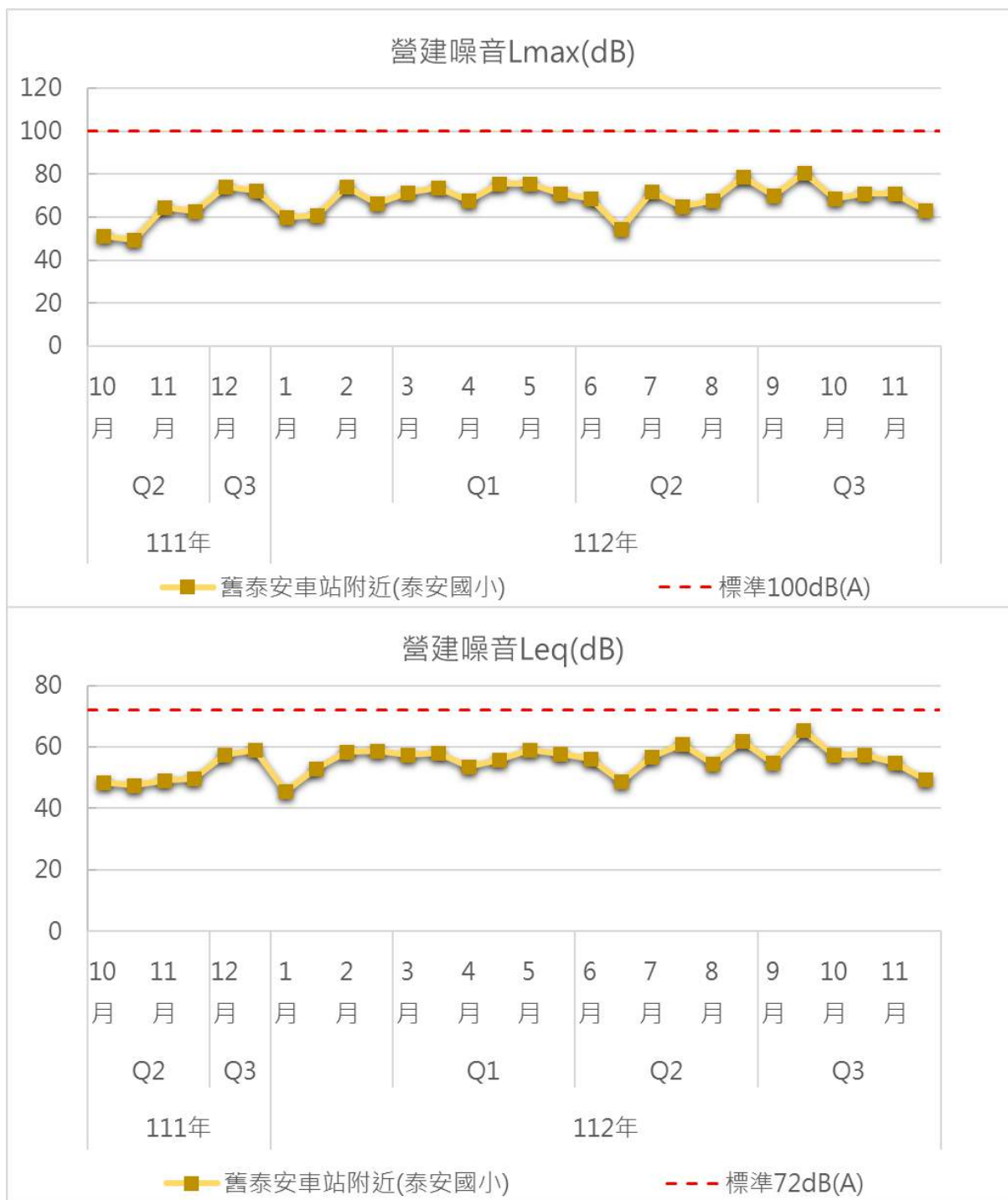
圖3.1.1-16 舊泰安車站附近(泰安國小)測站歷次營建噪音監測結果變化情形
