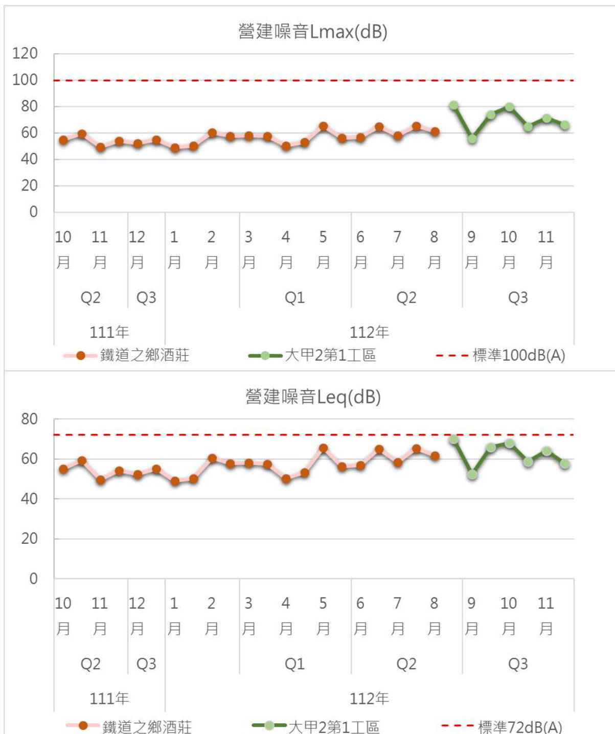
圖3.1.1-19 鐵道之鄉酒莊測站及大甲2第1工區測站歷次營建噪音監測結果變化情形
