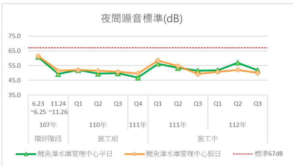
圖3.1.1-2 歷次鯉魚潭水庫管理中心測站噪音監測結果變化情形
