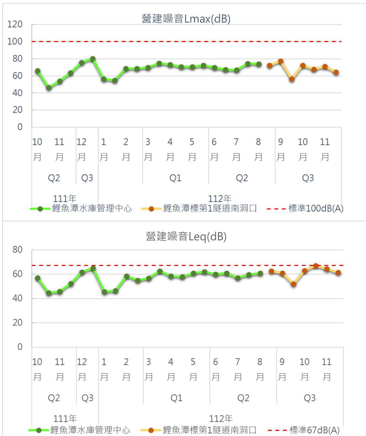
圖3.1.1-14 鯉魚潭水庫管理中心測站及鯉魚潭及第1隧道南洞口測站歷次營建噪音監測結果變化情形
