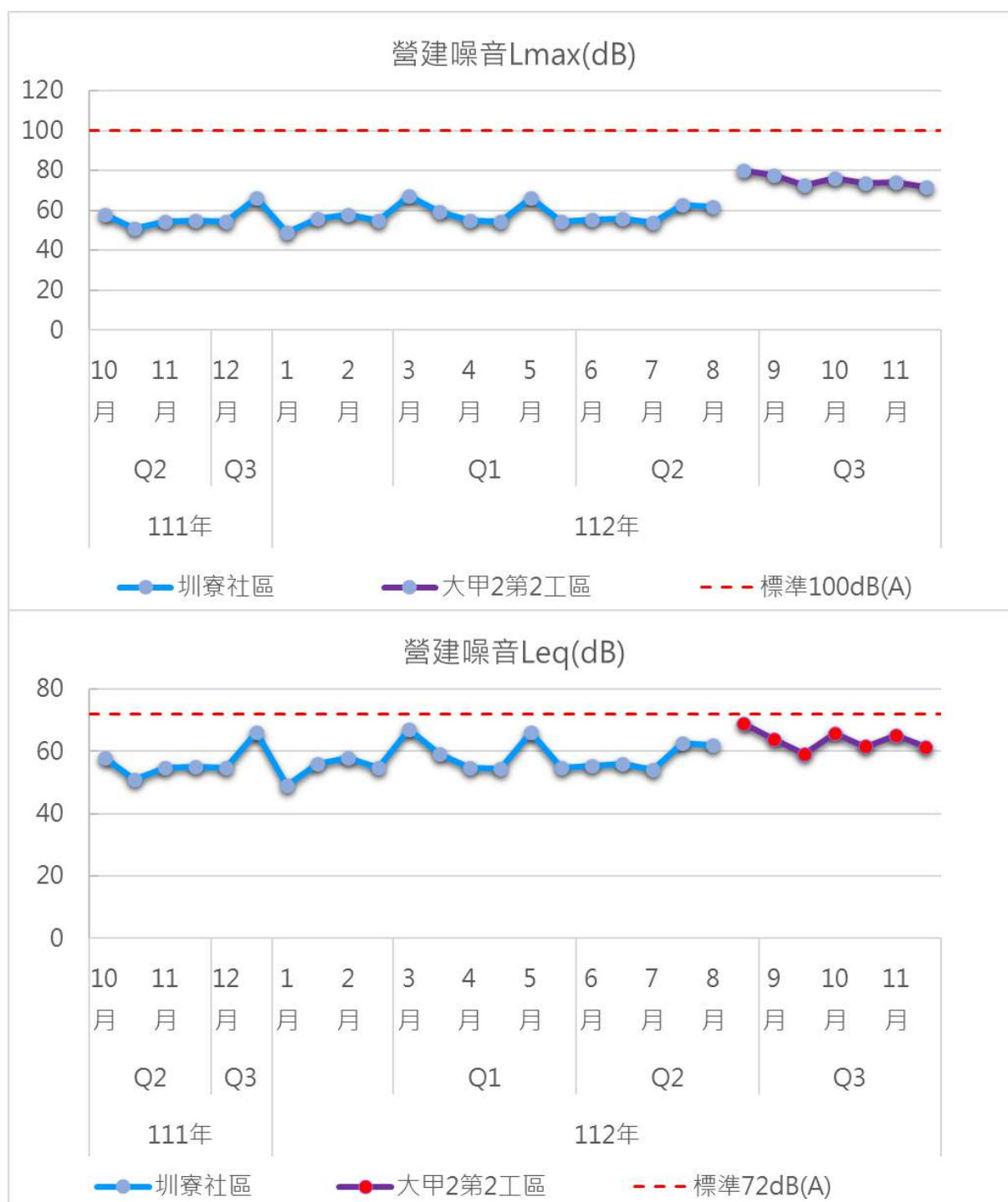
圖3.1.1-17 圳寮社區測站及大甲2第2工區測站歷次營建噪音監測結果變化情形
