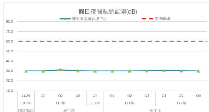
圖3.1.1-8 歷次鯉魚潭水庫管理中心測站振動監測結果變化情形
