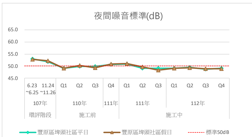
圖3.1.1-7 歷次豐原區埤頭社區測站噪音監測結果變化情形
