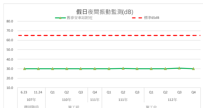
圖3.1.1-9 歷次舊泰安車站附近測站振動監測結果變化情形
