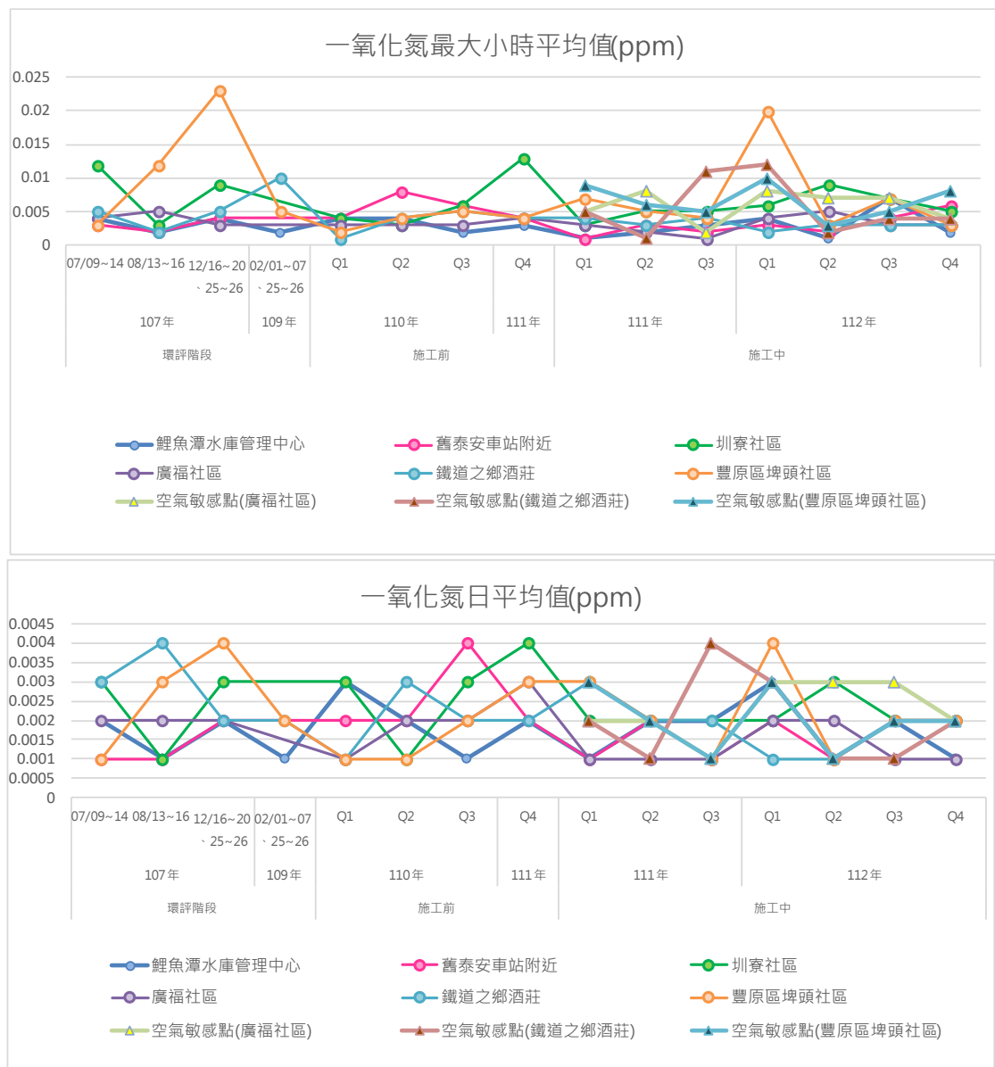
圖3.1.1-1 歷次空氣品質監測結果變化情形(續1)
