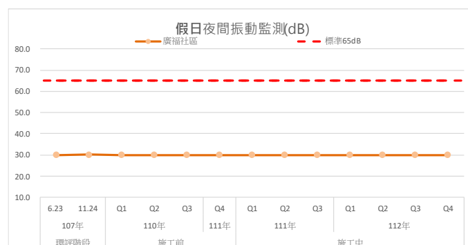
圖3.1.1-11 歷次廣福社區測站振動監測結果變化情形
