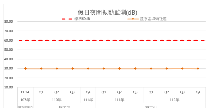
圖3.1.1-13 歷次豐原區埤頭社區測站振動監測結果變化情形
