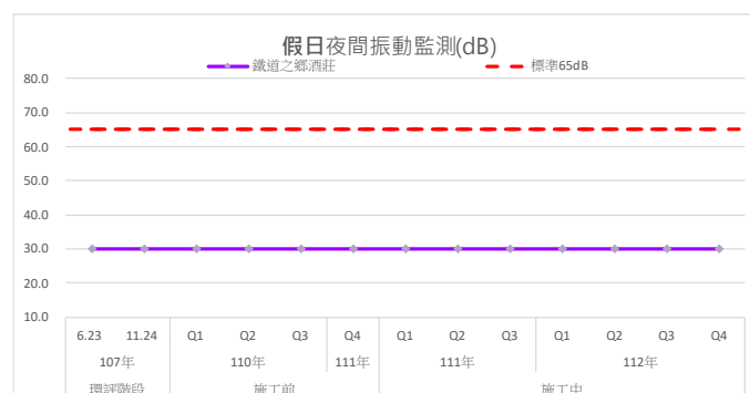
圖3.1.1-12 歷次鐵道之鄉酒莊測站振動監測結果變化情形
