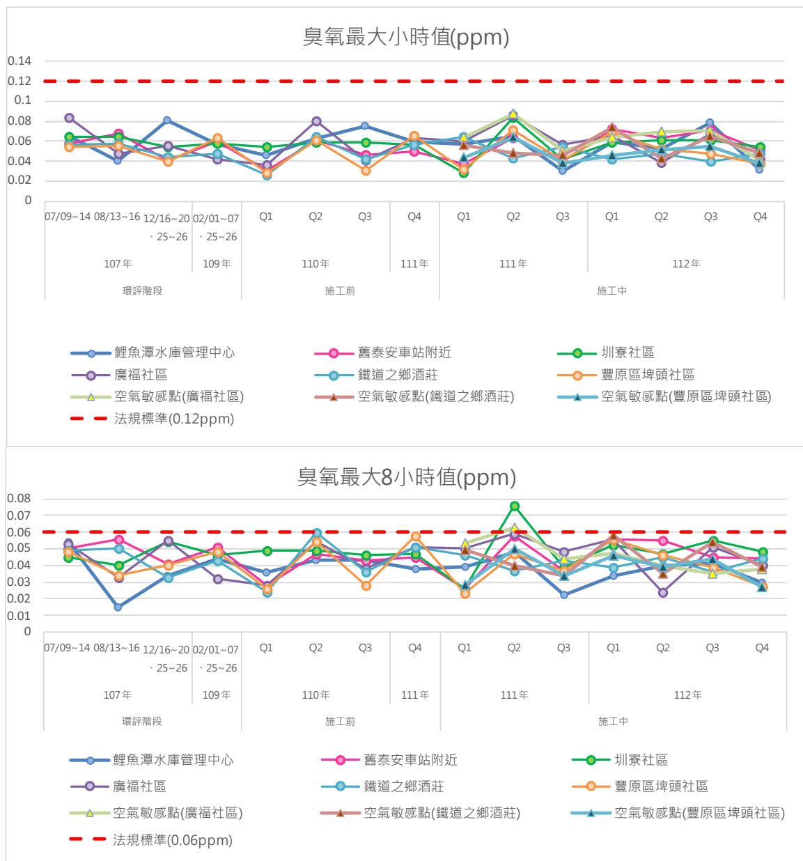
圖3.1.1-1 歷次空氣品質監測結果變化情形(續2)
