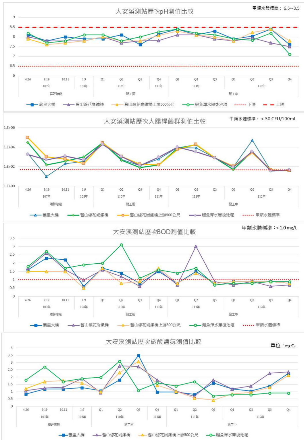
圖 3.1.1-20 歷次河川水質監測結果變化情形(大安溪測站)
