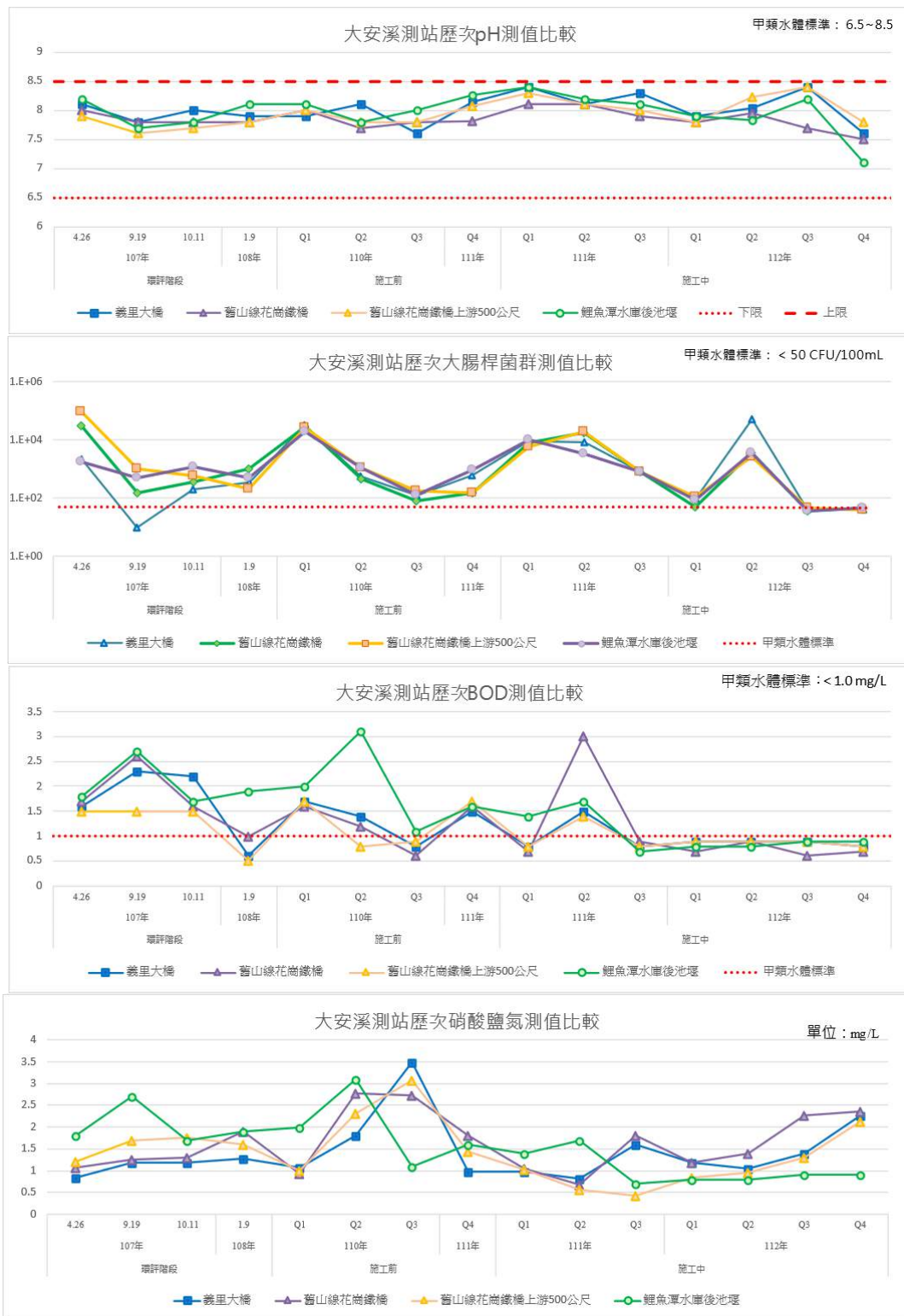
圖3.1.1-20 歷次河川水質監測結果變化情形(大安溪測站) (續1)
