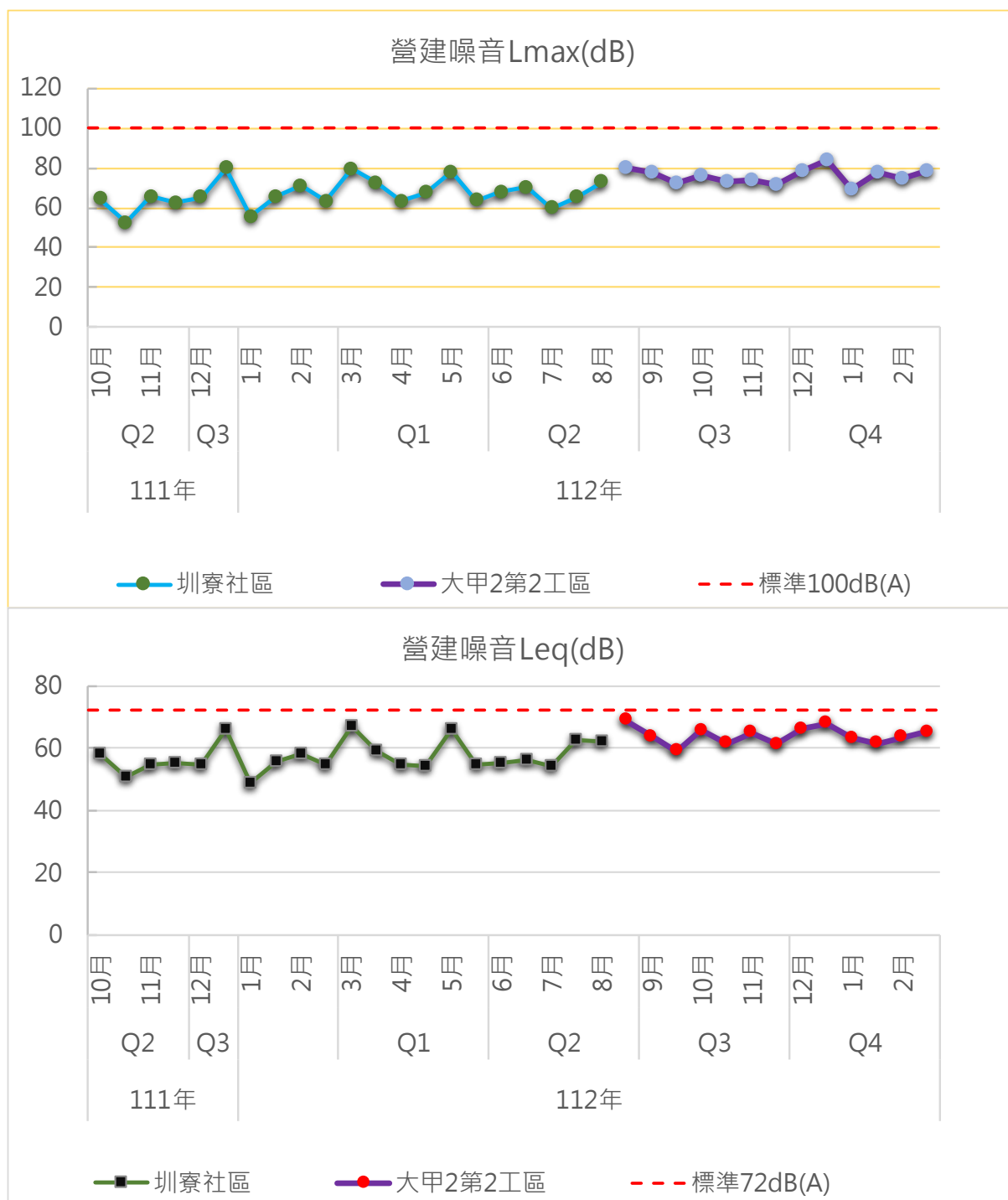
圖3.1.1-17 圳寮社區測站及大甲2第2工區測站歷次營建噪音監測結果變化情形
