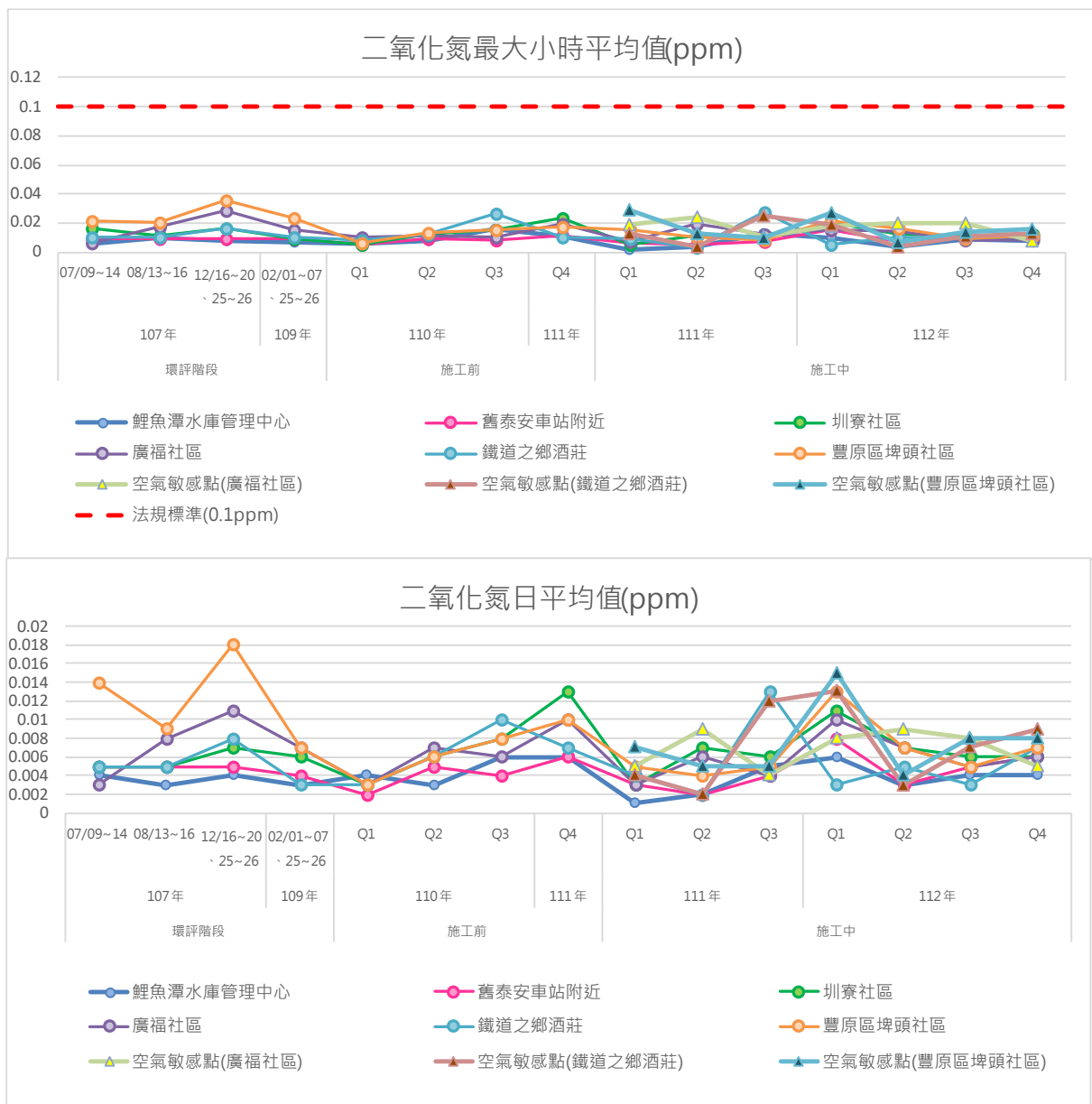
圖3.1.1-1 歷次空氣品質監測結果變化情形(續5)
