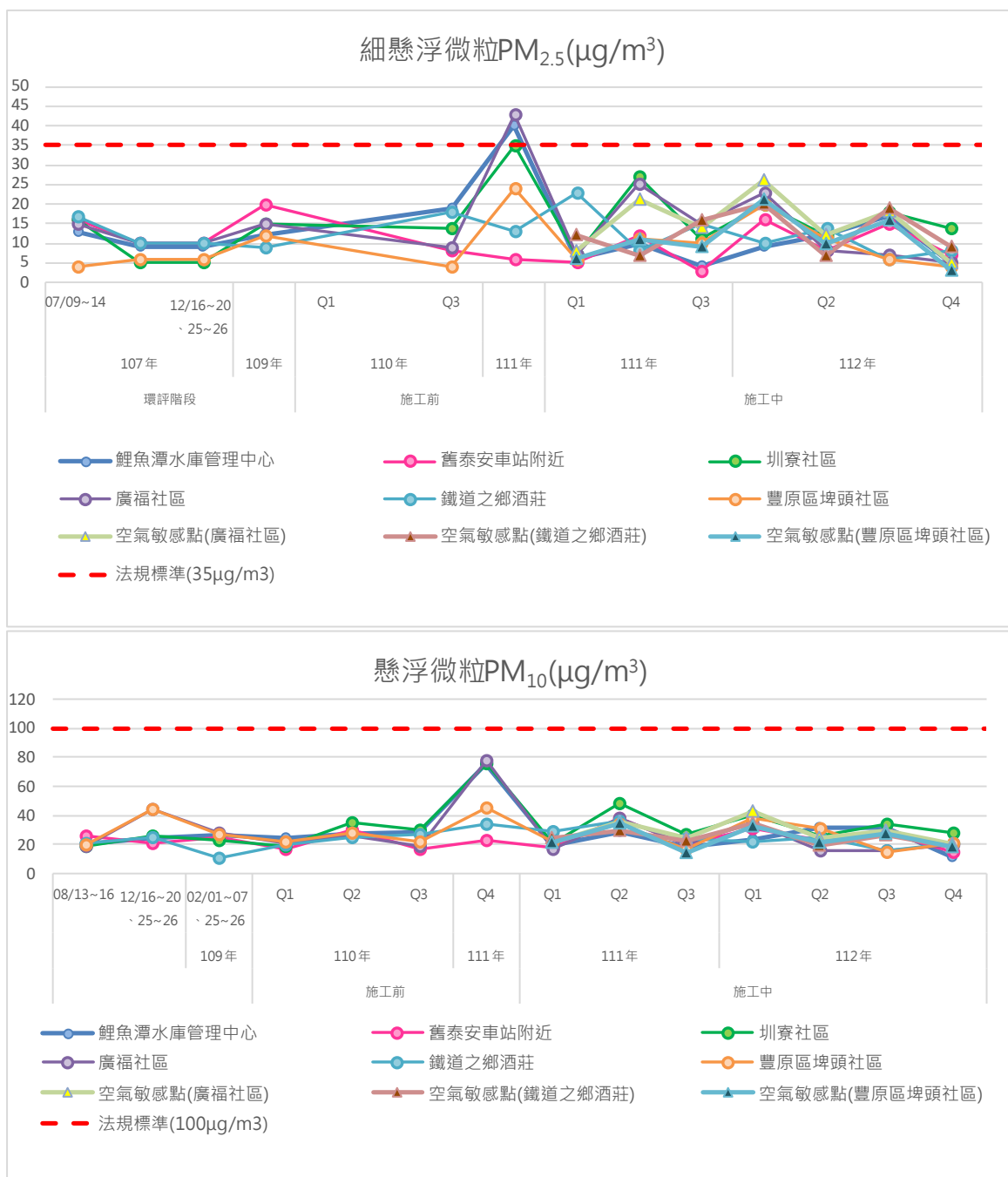
圖3.1.1-1 歷次空氣品質監測結果變化情形(續3)
