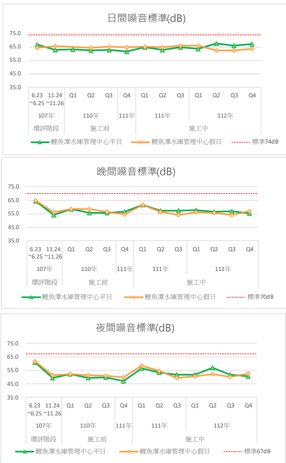
圖3.1.1-2 歷次鯉魚潭水庫管理中心測站噪音監測結果變化情形
