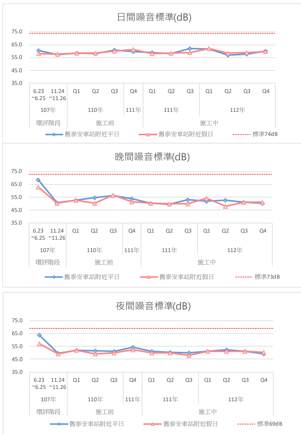
圖3.1.1-3 歷次舊泰安車站附近測站噪音監測結果變化情形
