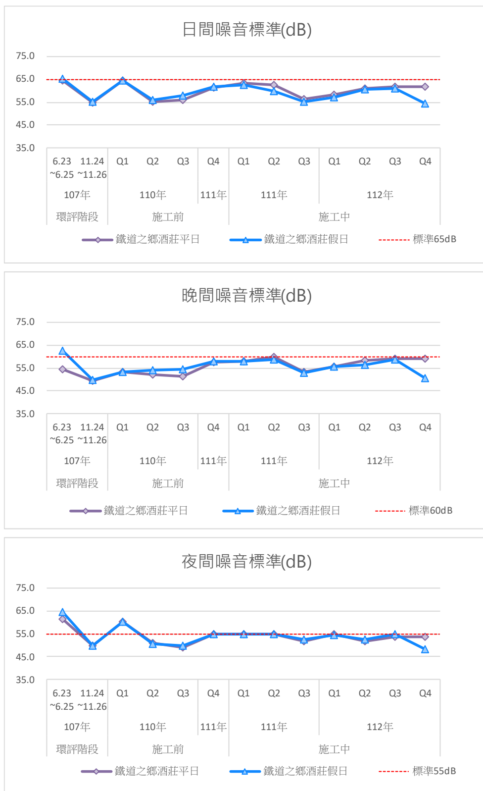
圖3.1.1-6 歷次鐵道之鄉酒莊測站噪音監測結果變化情形
