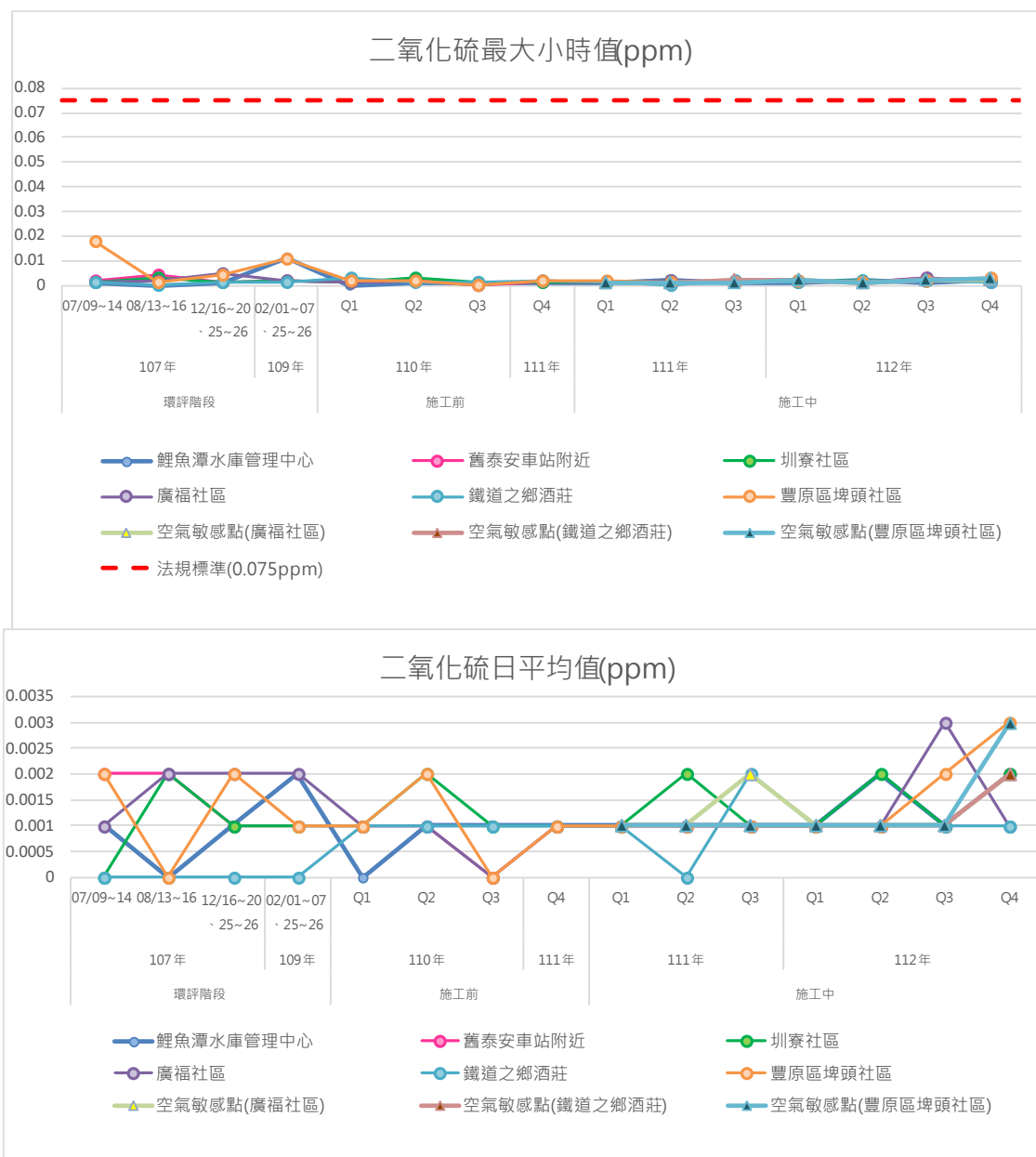
圖3.1.1-1 歷次空氣品質監測結果變化情形(續4)
