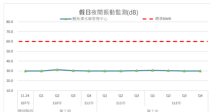
圖3.1.1-8 歷次鯉魚潭水庫管理中心測站振動監測結果變化情形
