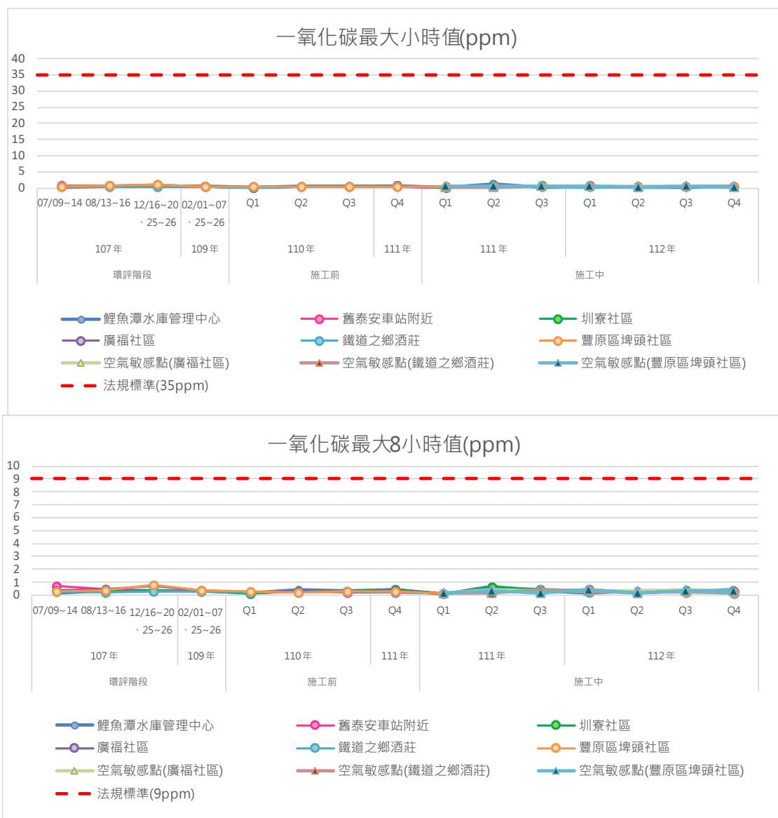
圖3.1.1-1 歷次空氣品質監測結果變化情形(續7)
