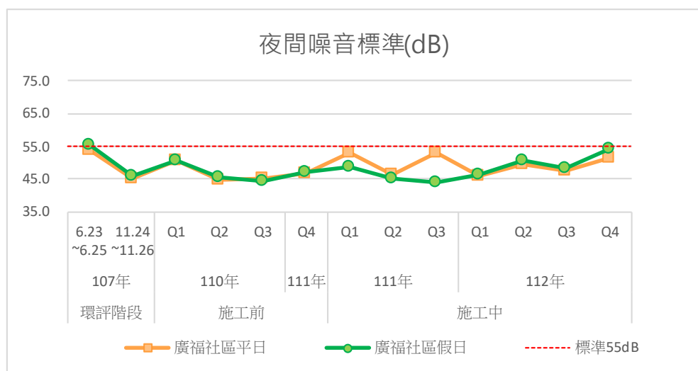
圖3.1.1-5 歷次廣福社區測站噪音監測結果變化情形
