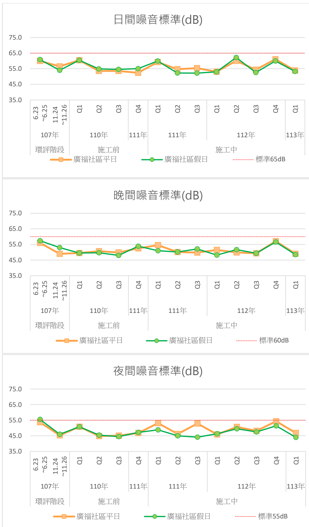
圖3.1.1-5 歷次廣福社區測站噪音監測結果變化情形
