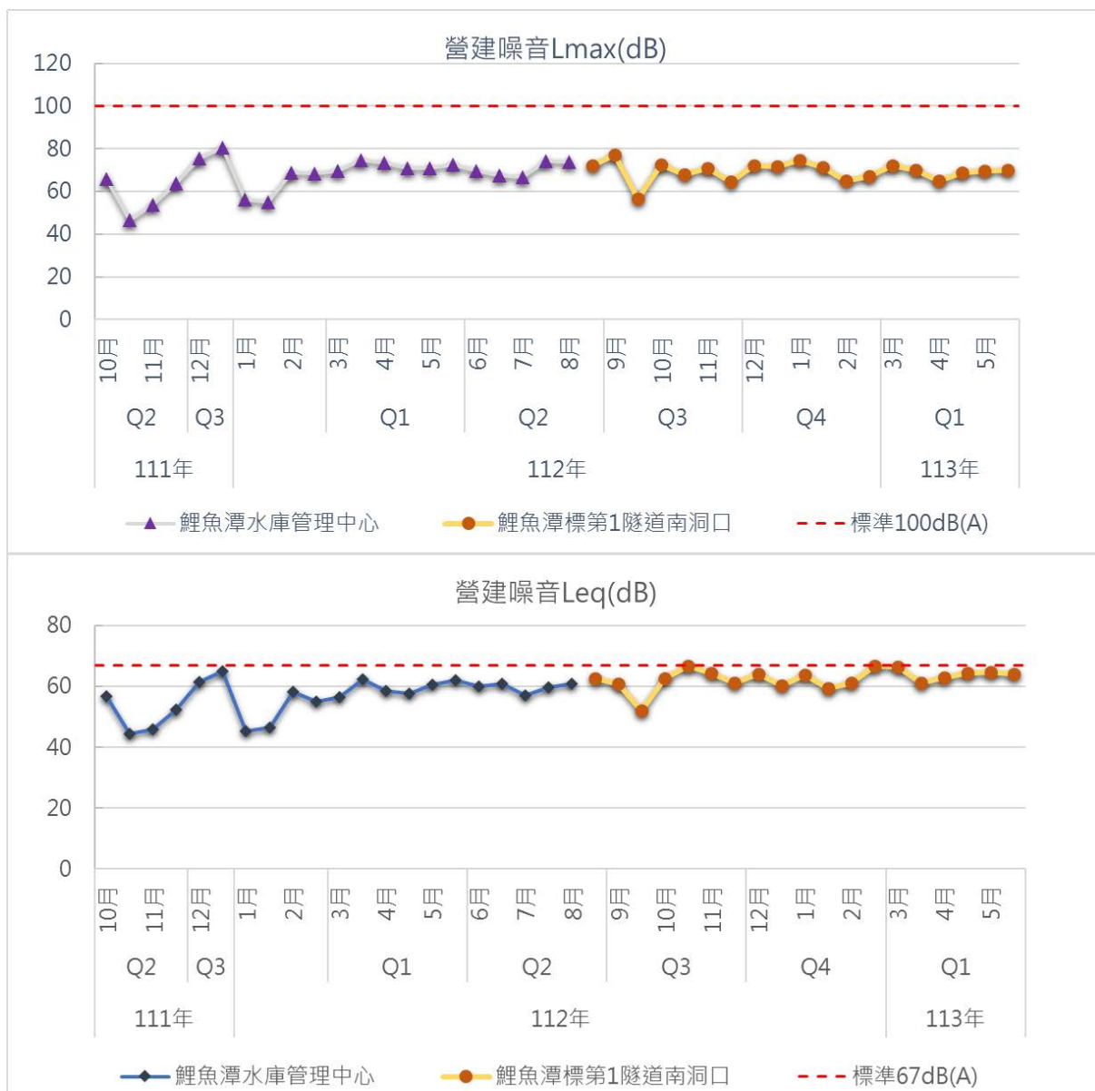
圖3.1.1-14 鯉魚潭水庫管理中心測站及鯉魚潭及第1隧道南洞口測站歷次營建噪音監測結果變化情形
