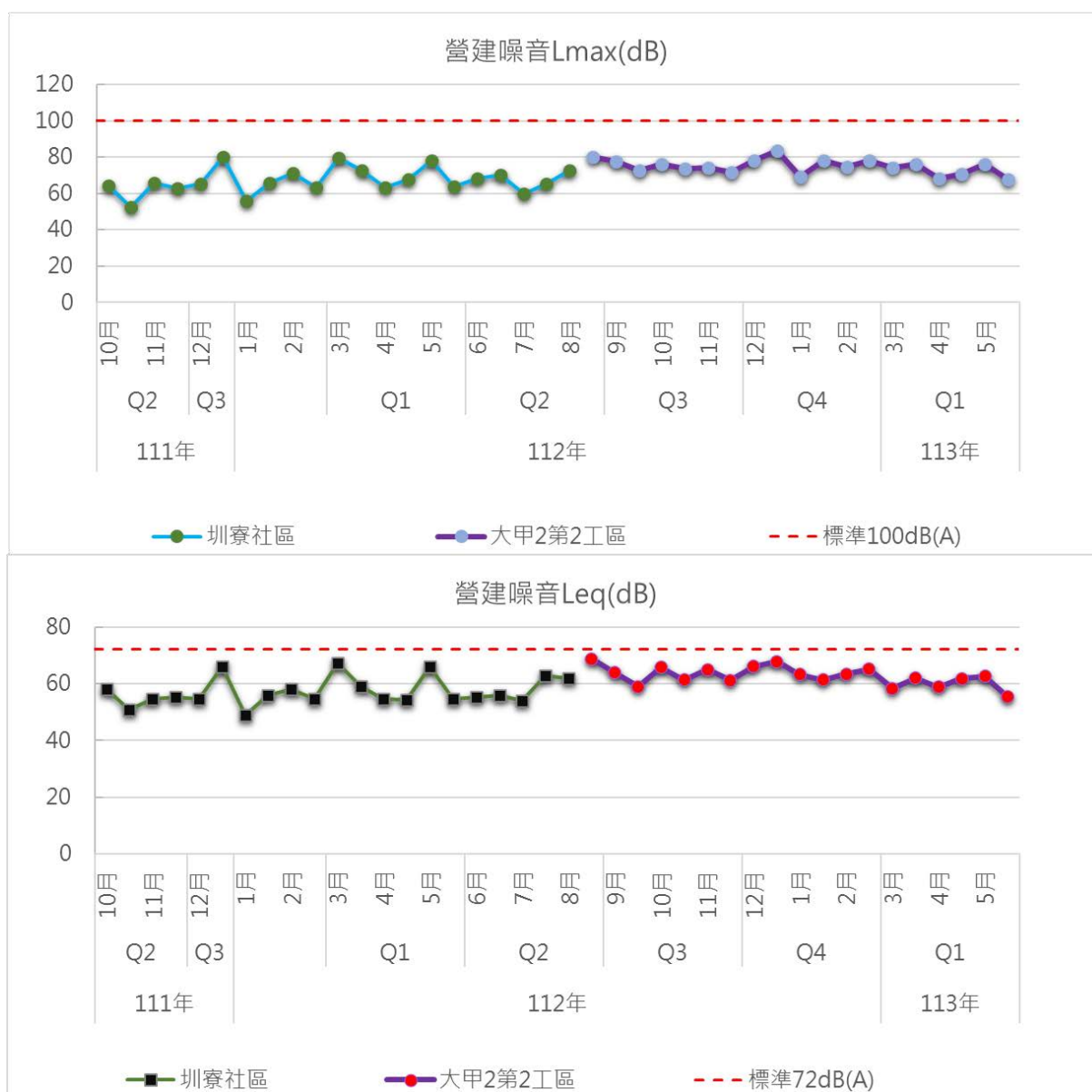
圖3.1.1-17 圳寮社區測站及大甲2第2工區測站歷次營建噪音監測結果變化情形
