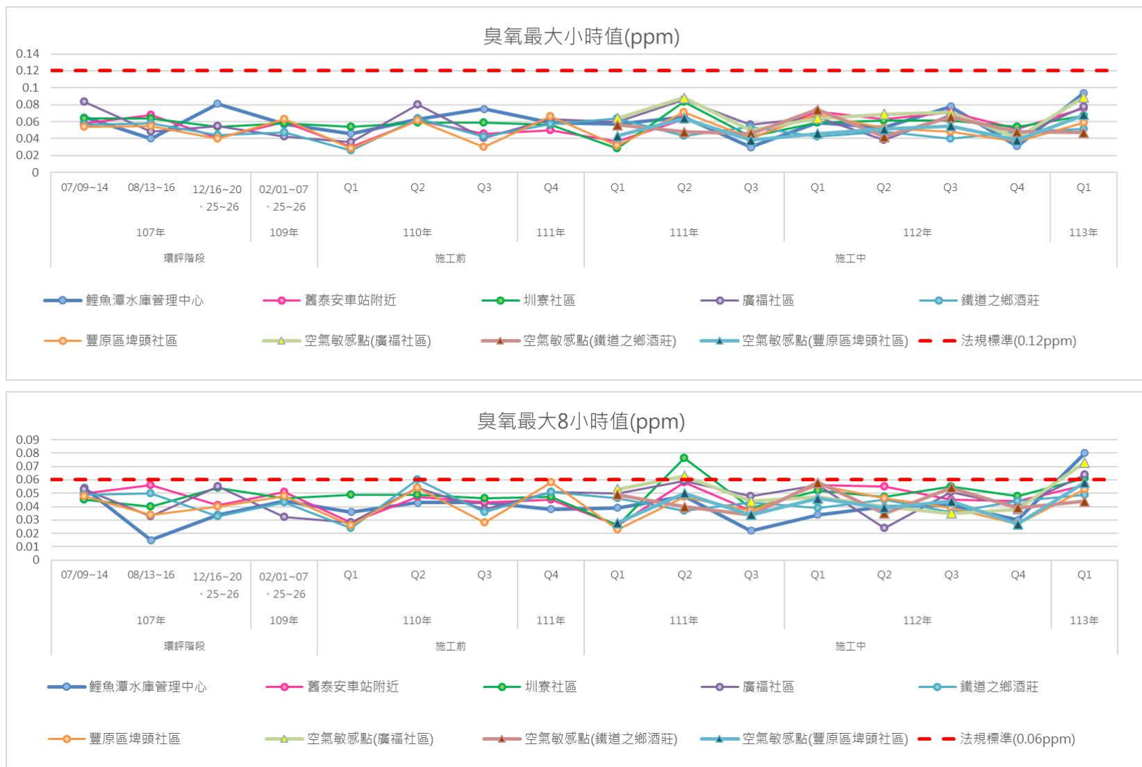
圖3.1.1-1 歷次空氣品質監測結果變化情形(續2)
