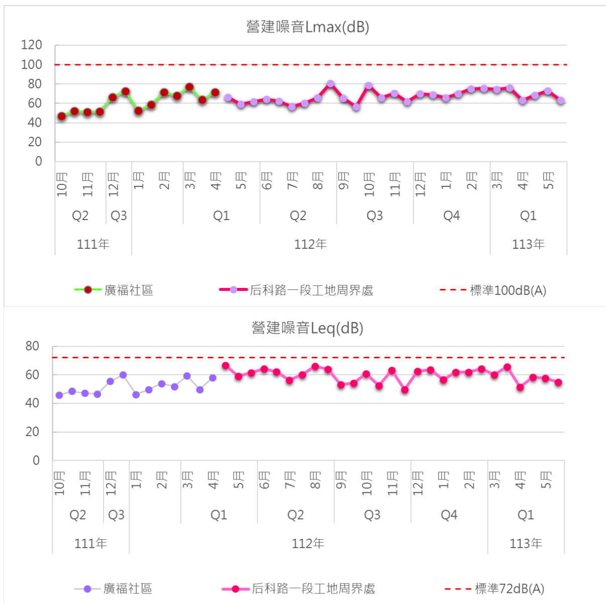
圖3.1.1-18 廣福社區測站及后科路一段工地周界處測站歷次營建噪音監測結果變化情形
