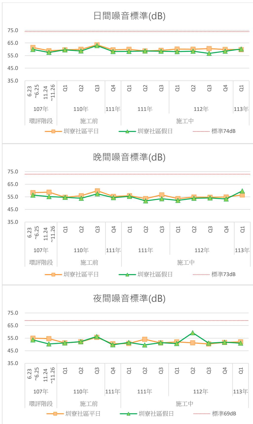
圖3.1.1-4 歷次圳寮社區測站噪音監測結果變化情形
