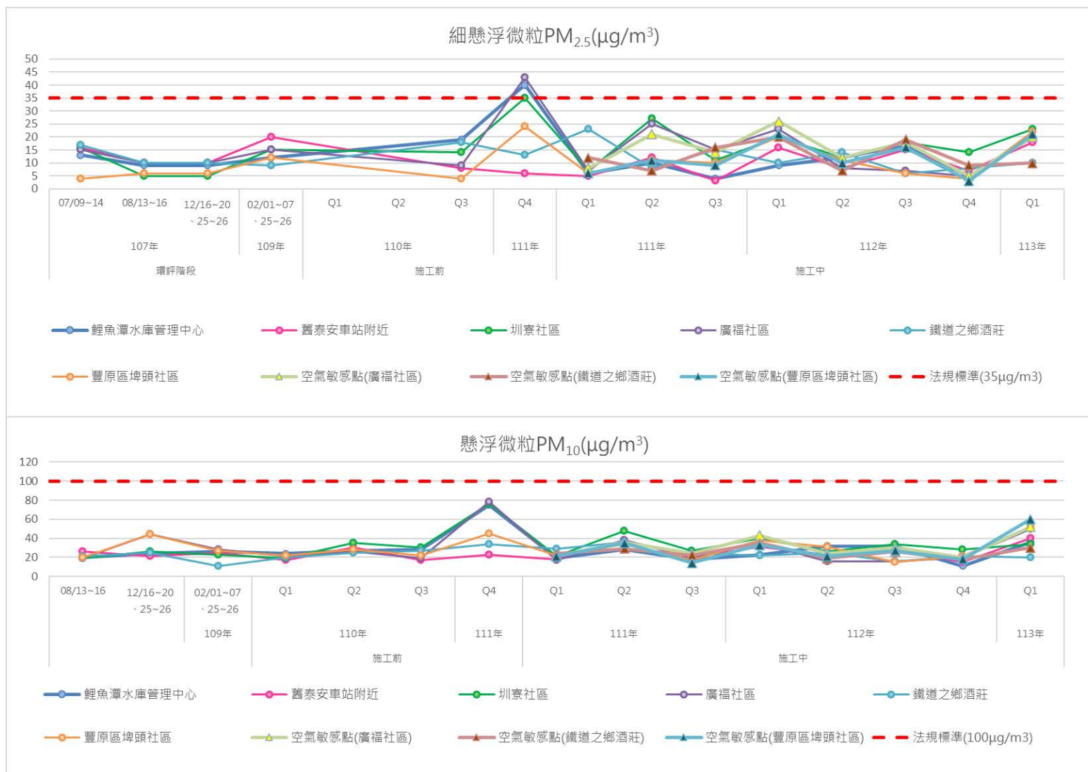
圖3.1.1-1 歷次空氣品質監測結果變化情形(續3)
