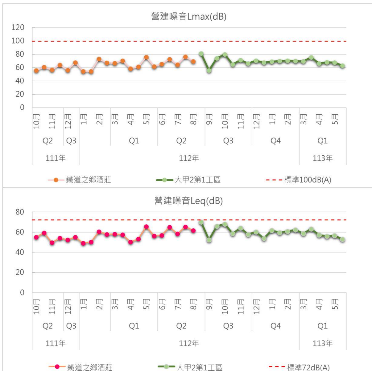
圖3.1.1-19 鐵道之鄉酒莊測站及大甲2第1工區測站歷次營建噪音監測結果變化情形
