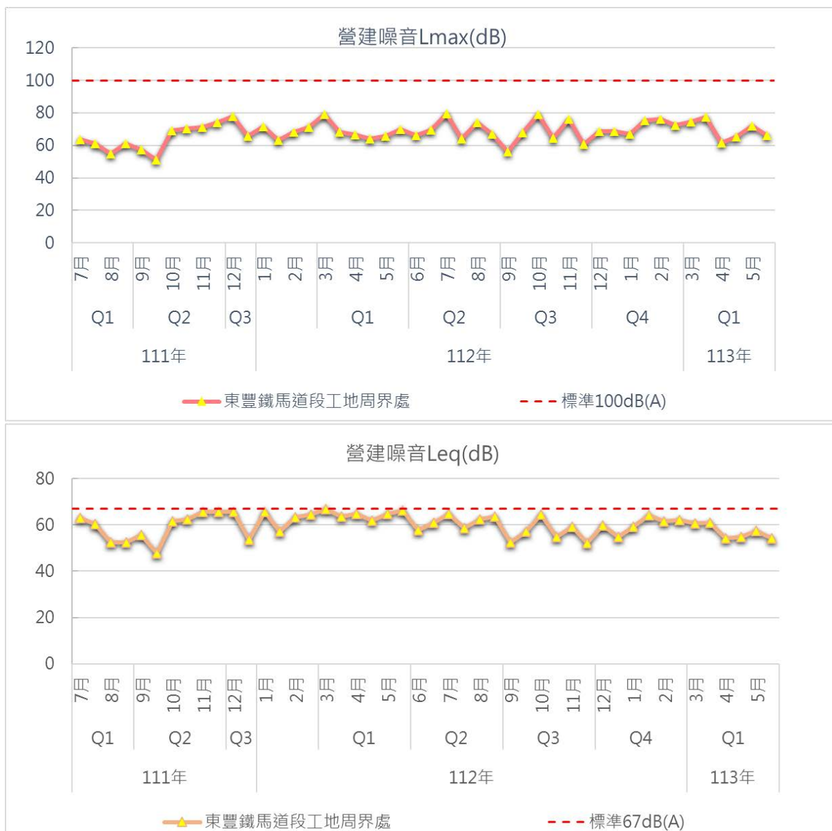
圖3.1.1-15 東豐鐵馬道段工地周界處測站歷次營建噪音監測結果變化情形
