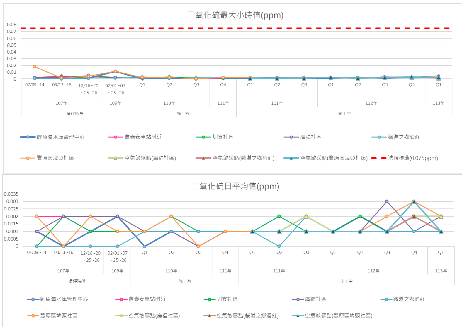
圖3.1.1-1 歷次空氣品質監測結果變化情形(續4)
