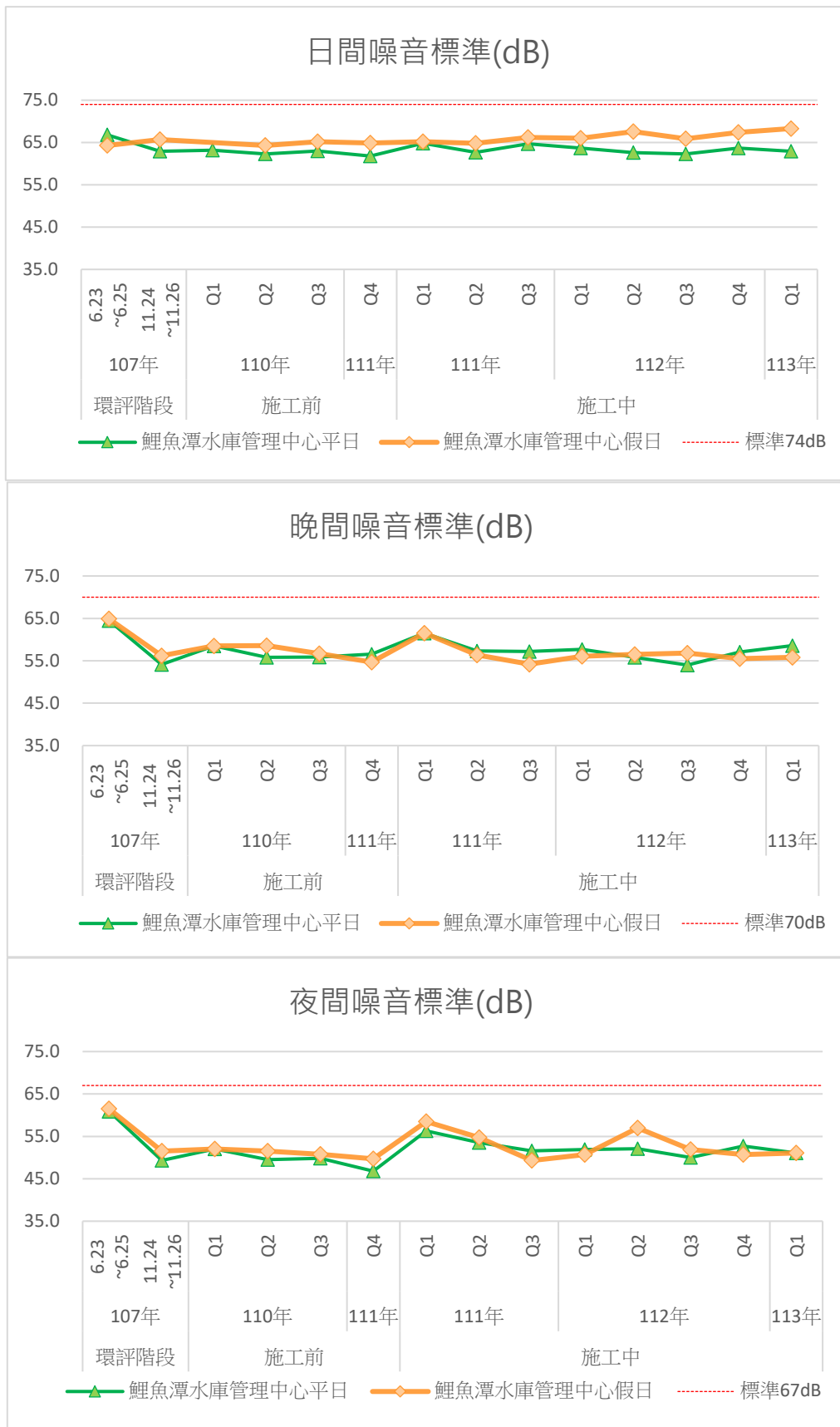
圖3.1.1-2 歷次鯉魚潭水庫管理中心測站噪音監測結果變化情形
