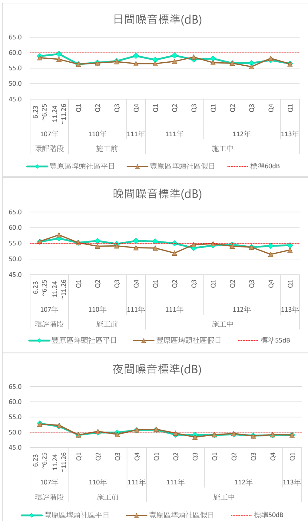
圖3.1.1-7 歷次豐原區埤頭社區測站噪音監測結果變化情形
