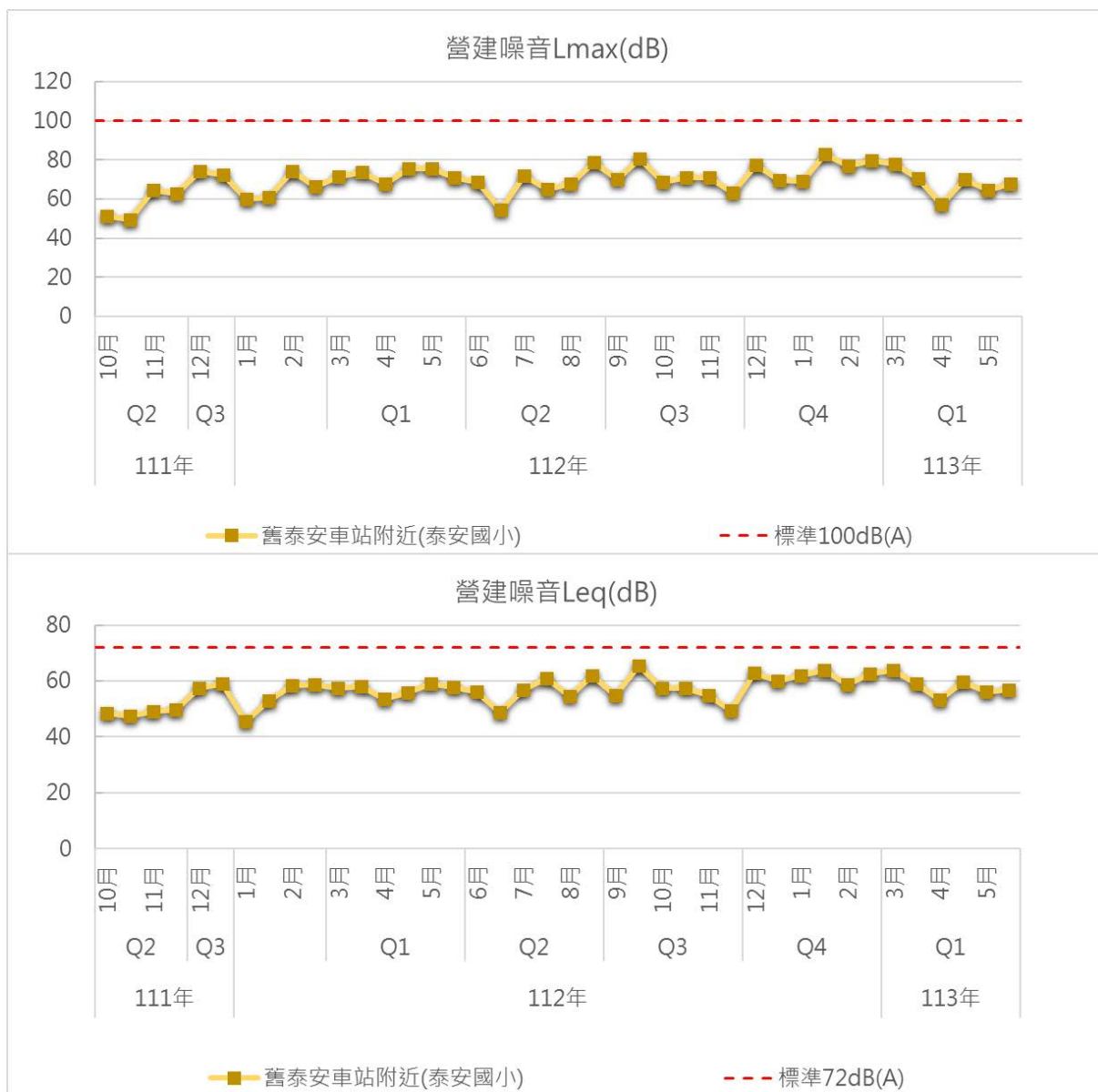
圖3.1.1-16 舊泰安車站附近(泰安國小)測站歷次營建噪音監測結果變化情形
