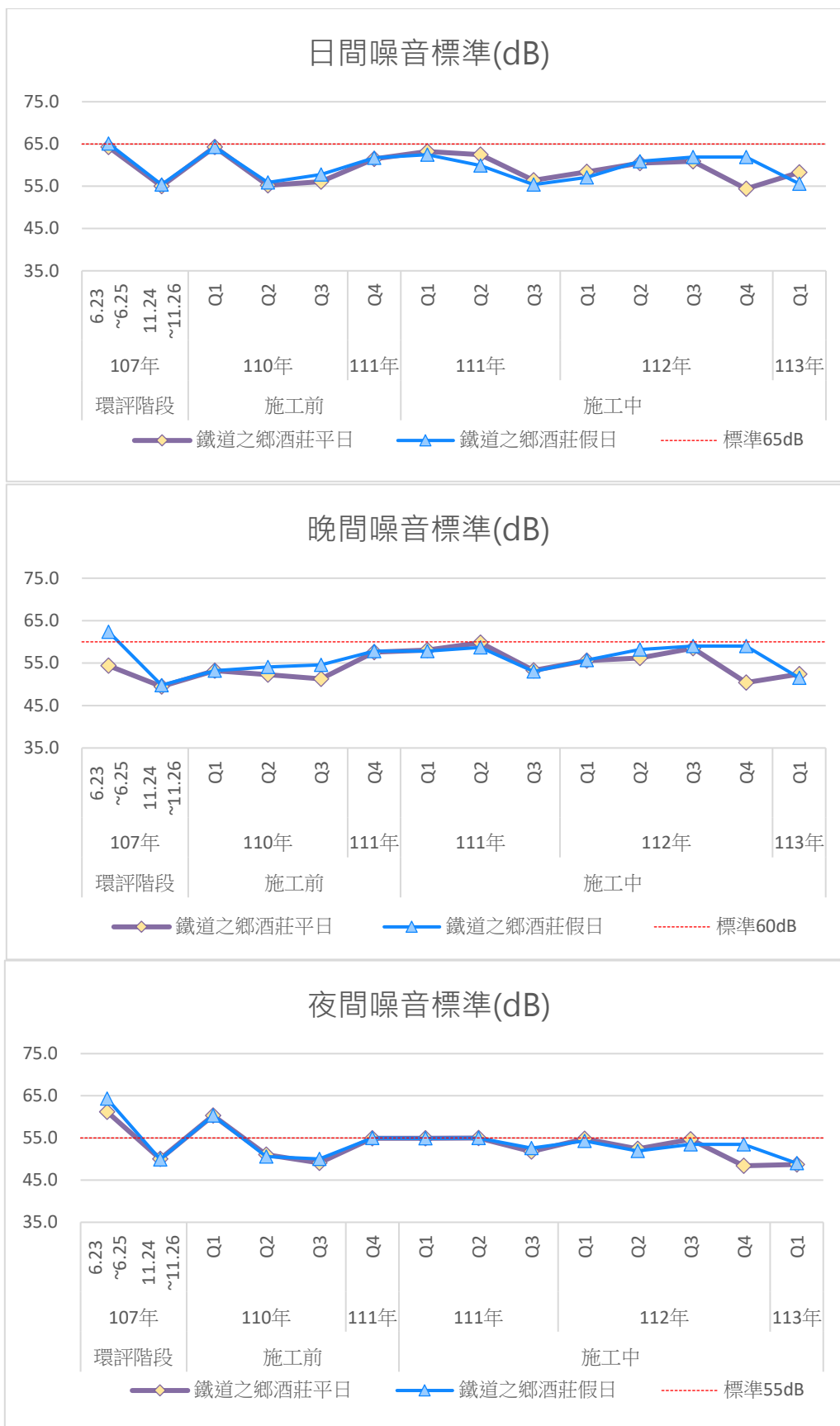
圖3.1.1-6 歷次鐵道之鄉酒莊測站噪音監測結果變化情形
