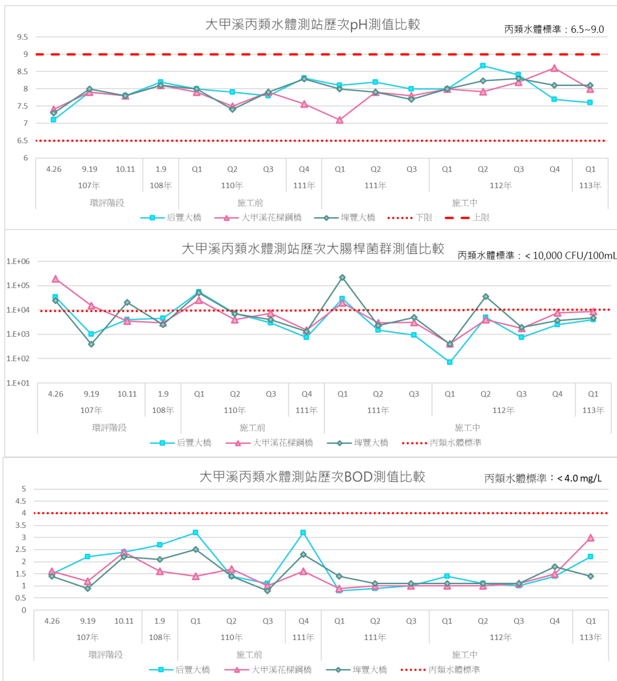
圖3.1.1-21 歷次河川水質監測結果變化情形(大甲溪丙類水體測站)
