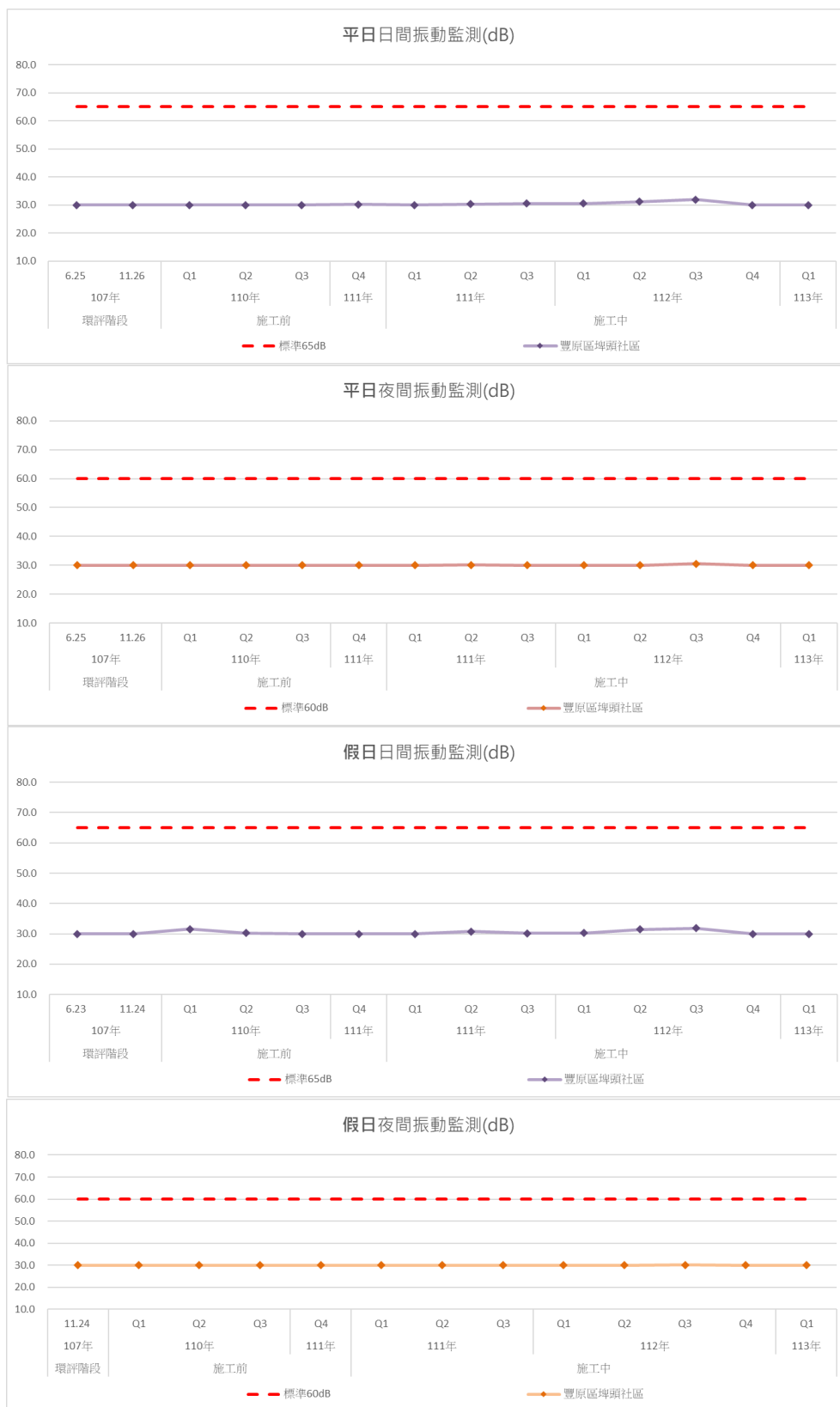
圖3.1.1-13 歷次豐原區埤頭社區測站振動監測結果變化情形
