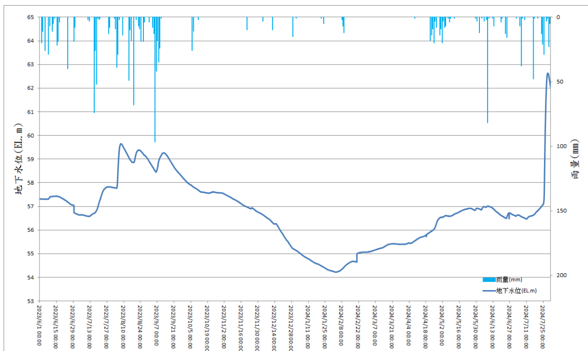
圖 10 舊正(1)觀測井地下水位歷線圖
