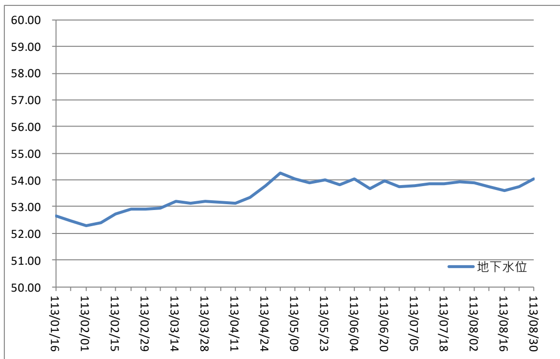
圖 4 BH-3 觀測井地下水位歷線圖
