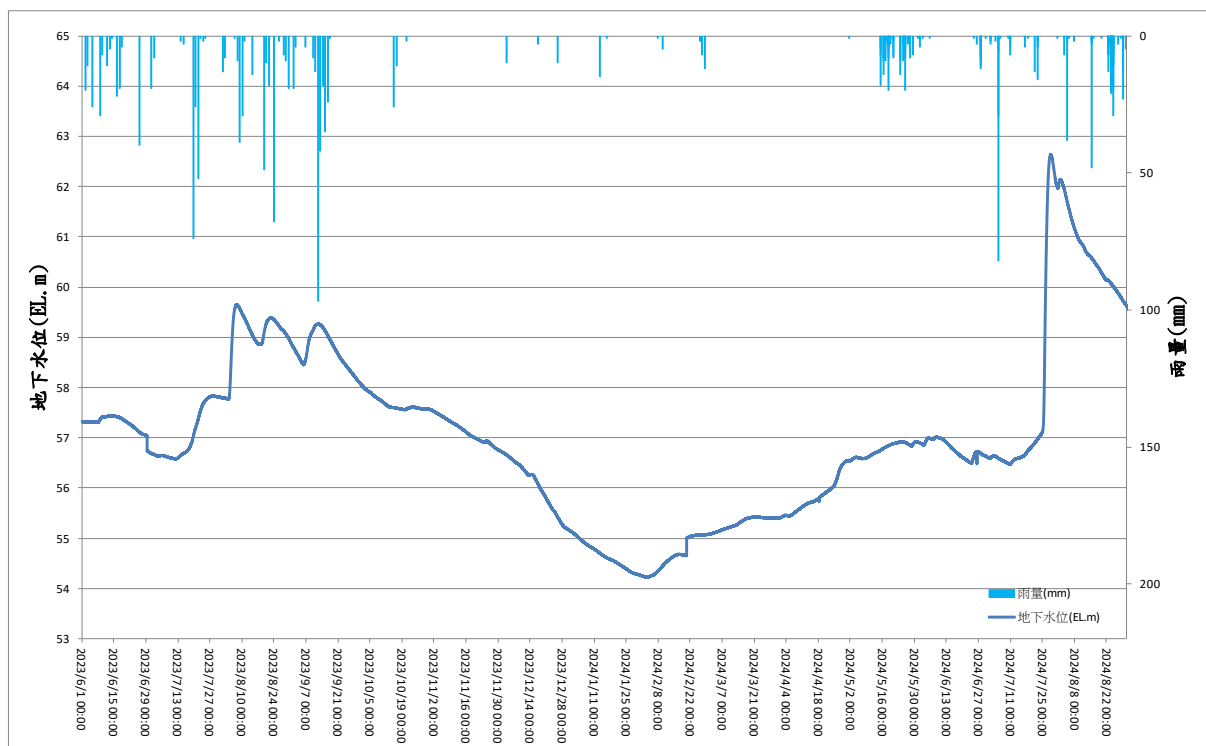
圖 10 舊正(1)觀測井地下水位歷線圖
