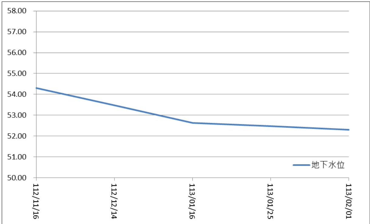
圖 4 BH-3 觀測井地下水位歷線圖
