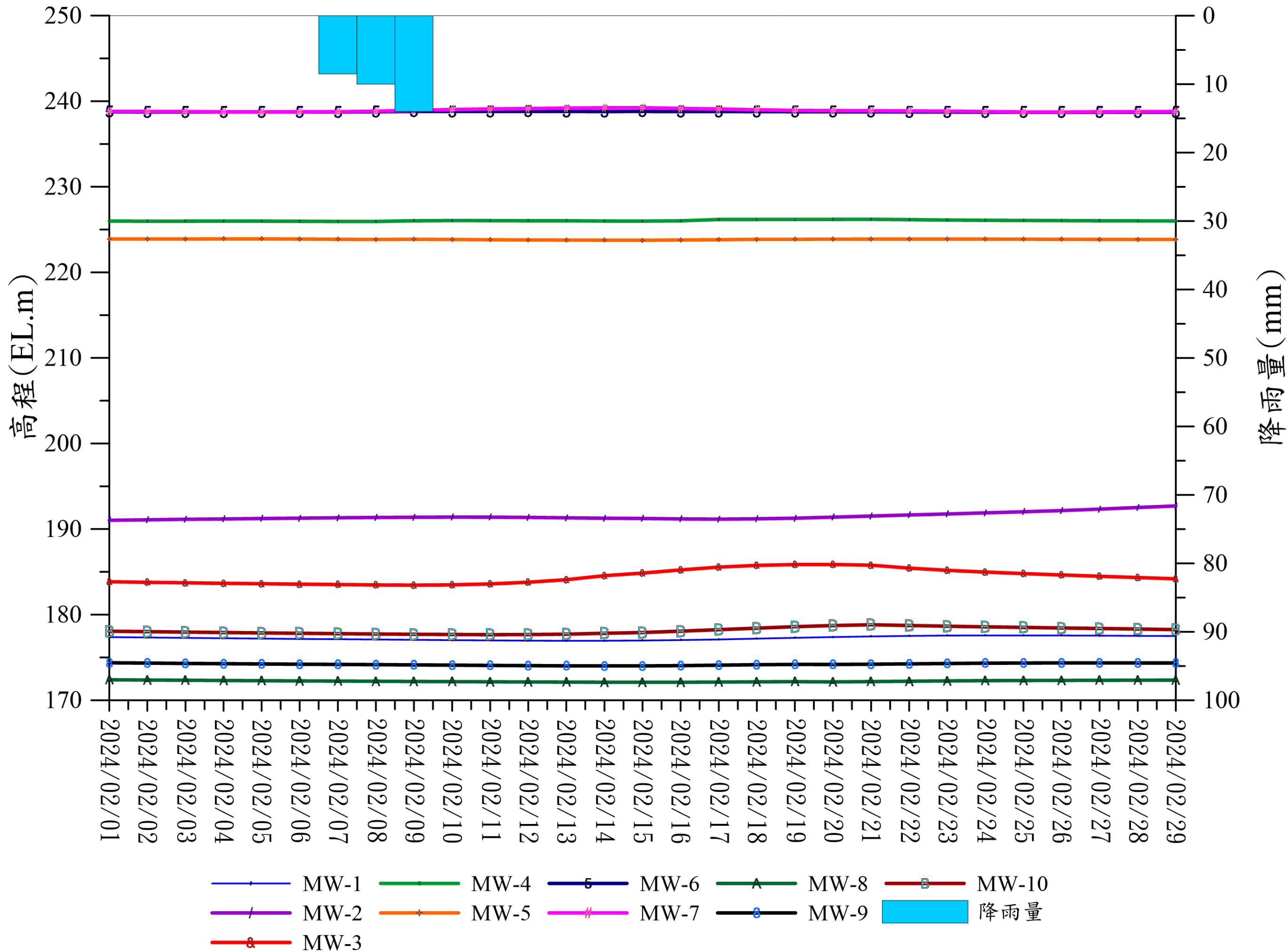
大安溪2024年2月之觀測地下水位-降雨量歷線圖
