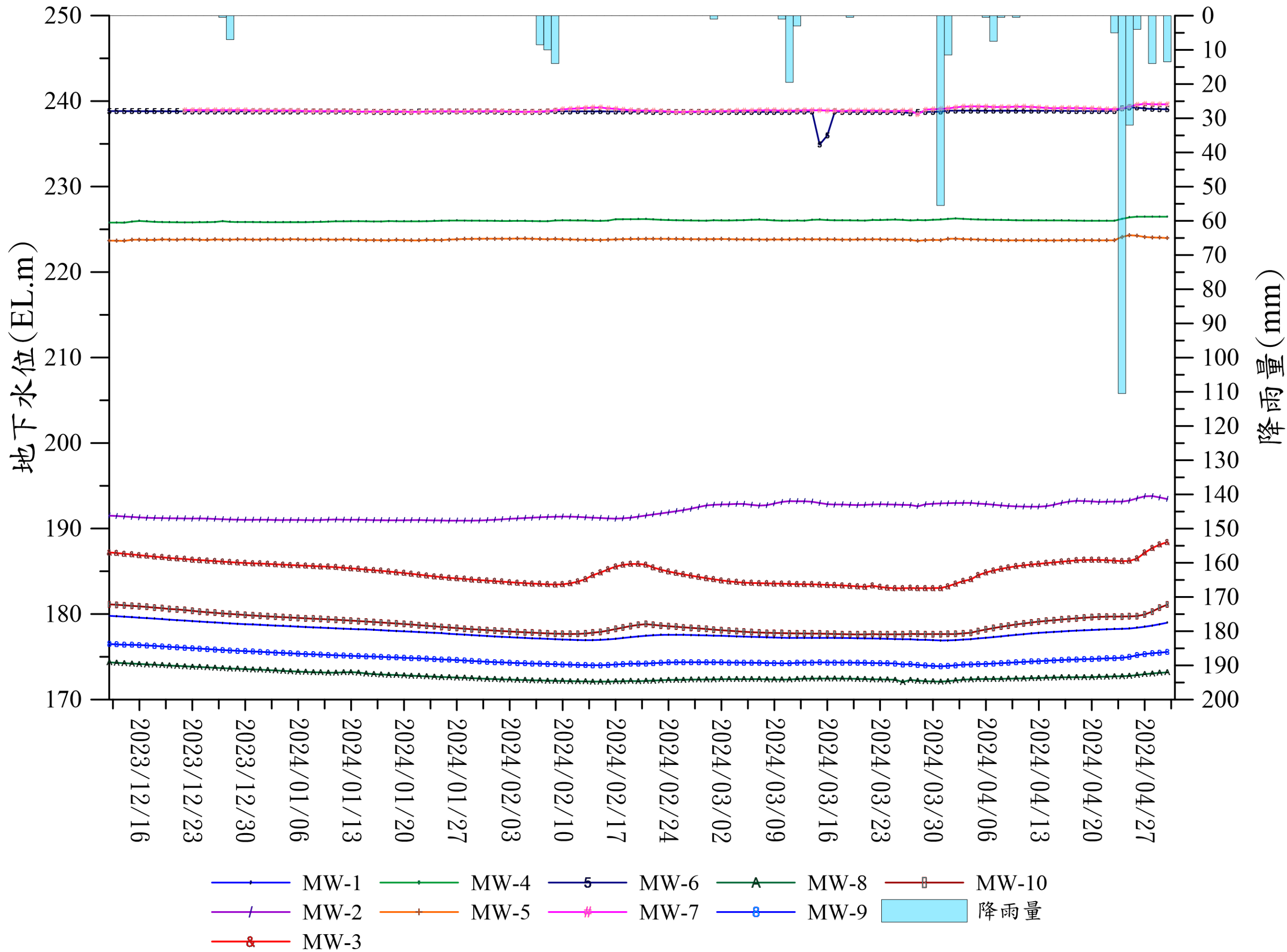
大安溪2023/12~2024/04之觀測地下水位-降雨量歷線圖
