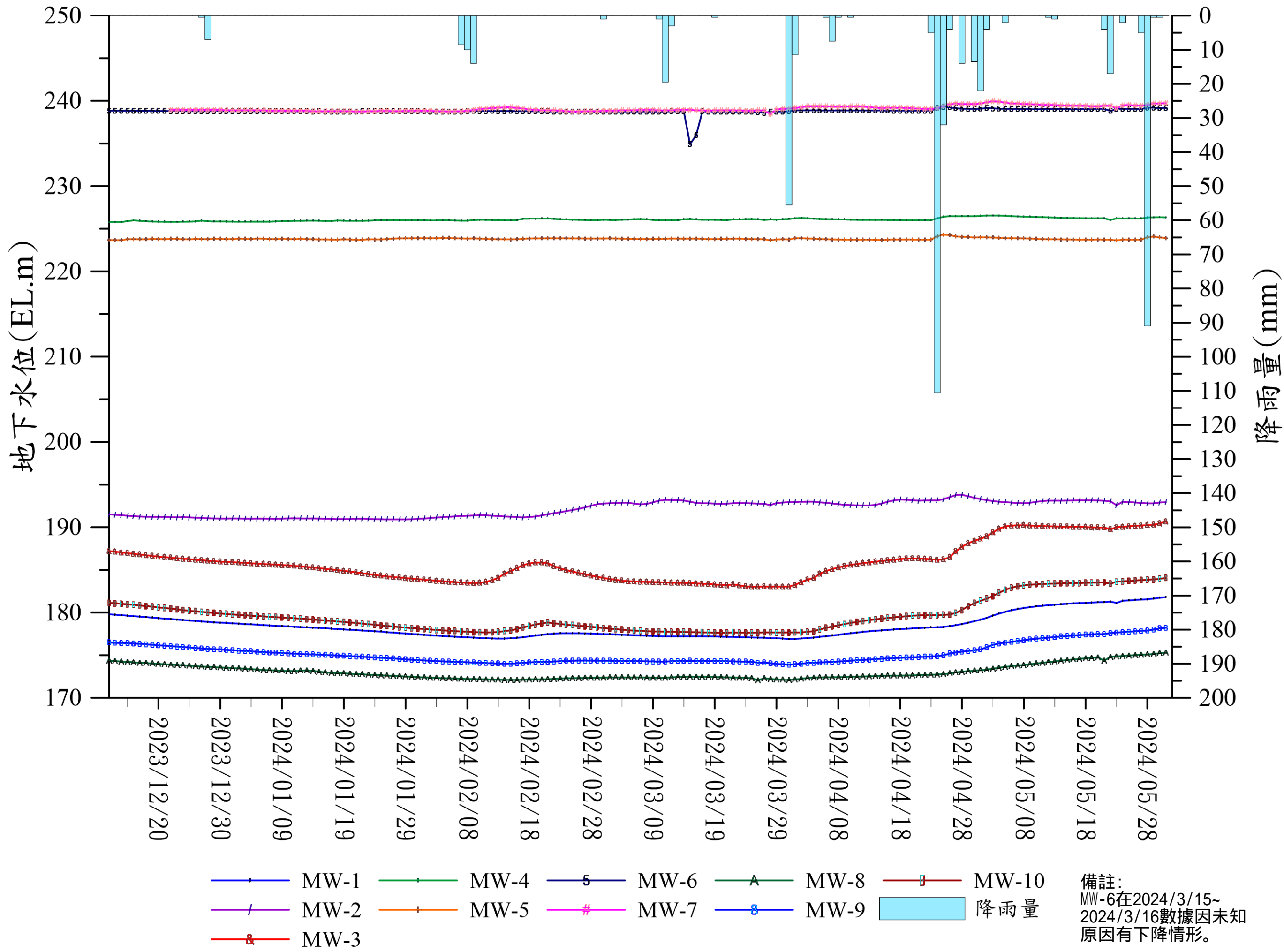
大安溪2023/12~2024/05之觀測地下水位-降雨量歷線圖
