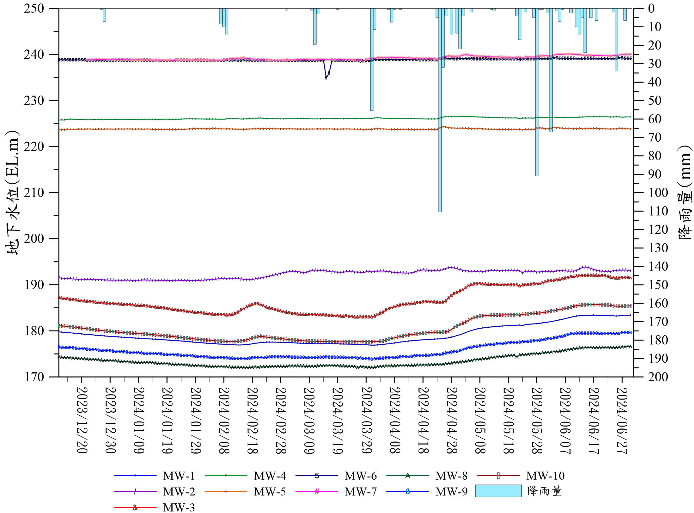
大安溪2023/12~2024/06之觀測地下水位-降雨量歷線圖
