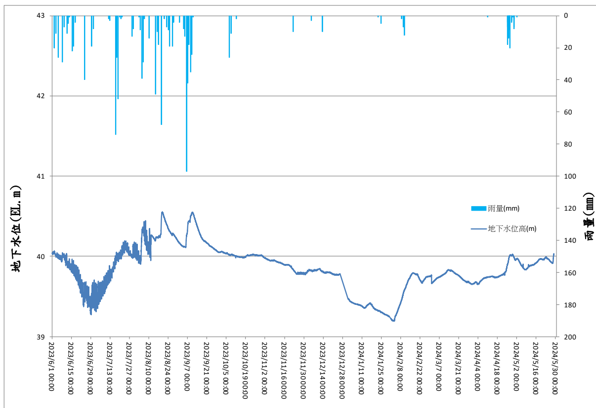
圖 8 溪岸(1)觀測井地下水位歷線圖
