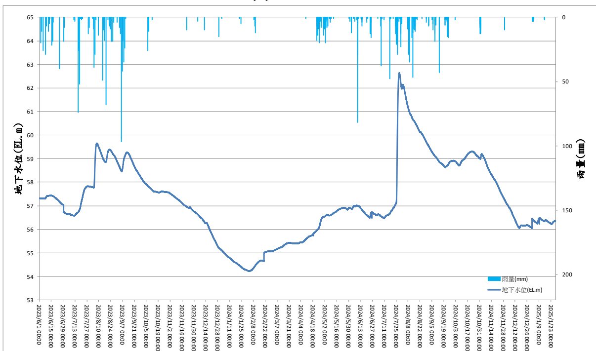
圖 7 舊正(1)觀測井地下水位歷線圖
