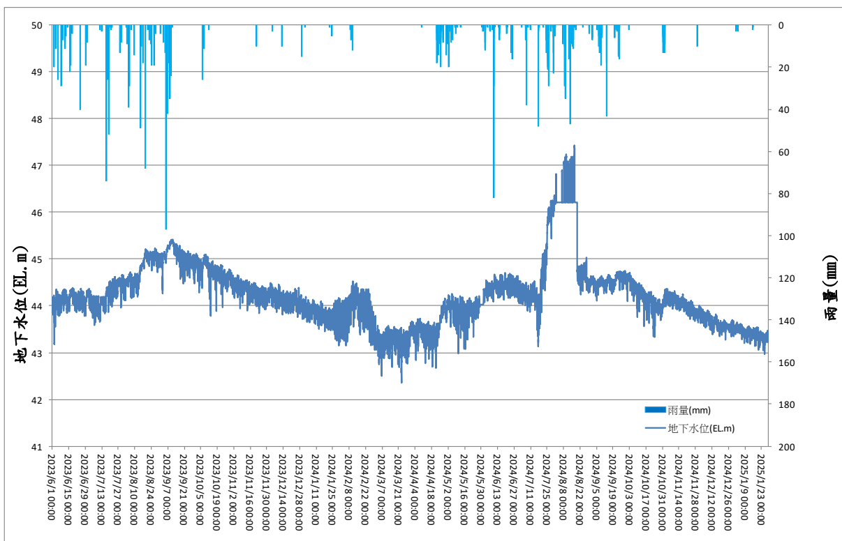
圖 6 霧峰(1)觀測井地下水位歷線圖
