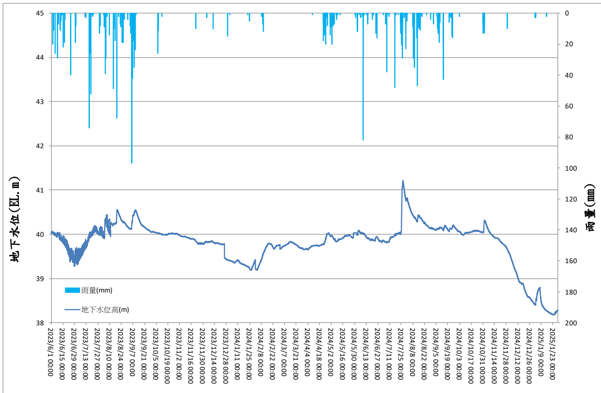
圖 5 溪岸(1)觀測井地下水位歷線圖
