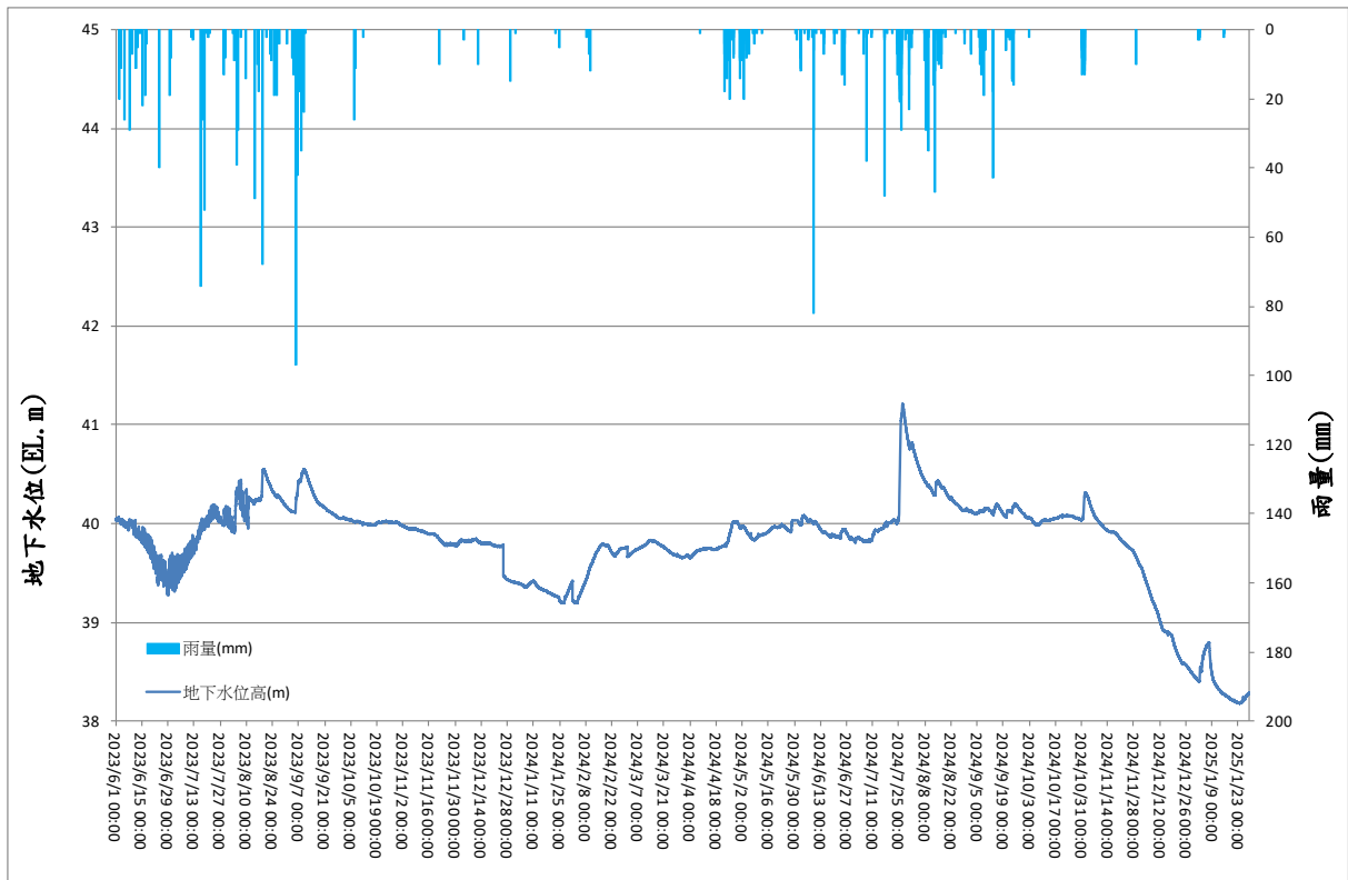
圖 8 草屯觀測井地下水位歷線圖
