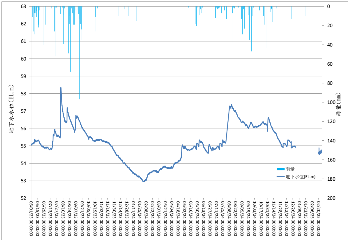
圖 6 BH-6 觀測井地下水位歷線圖
