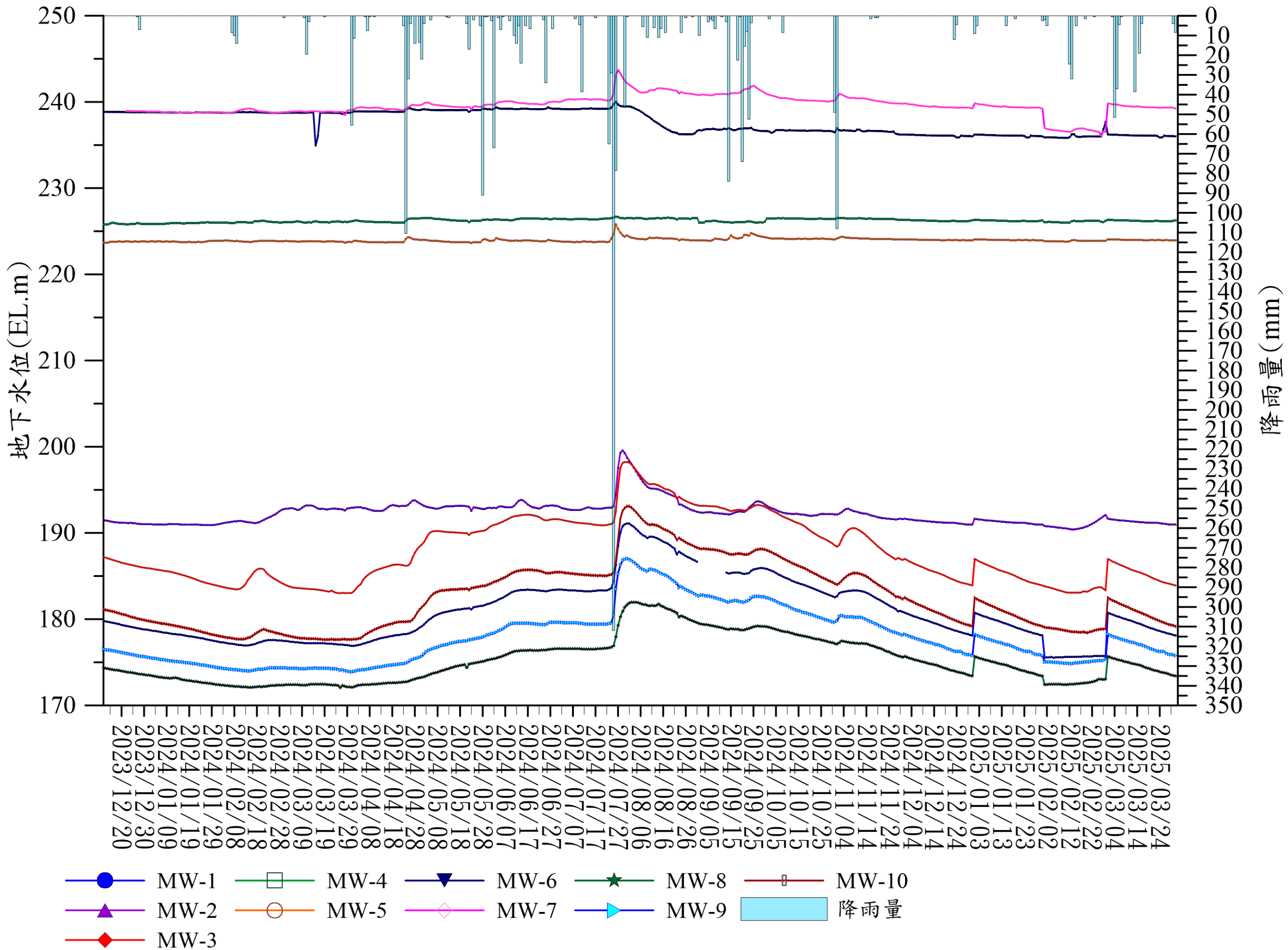
大安溪2023/12~2025/3之觀測地下水位-降雨量歷線圖
