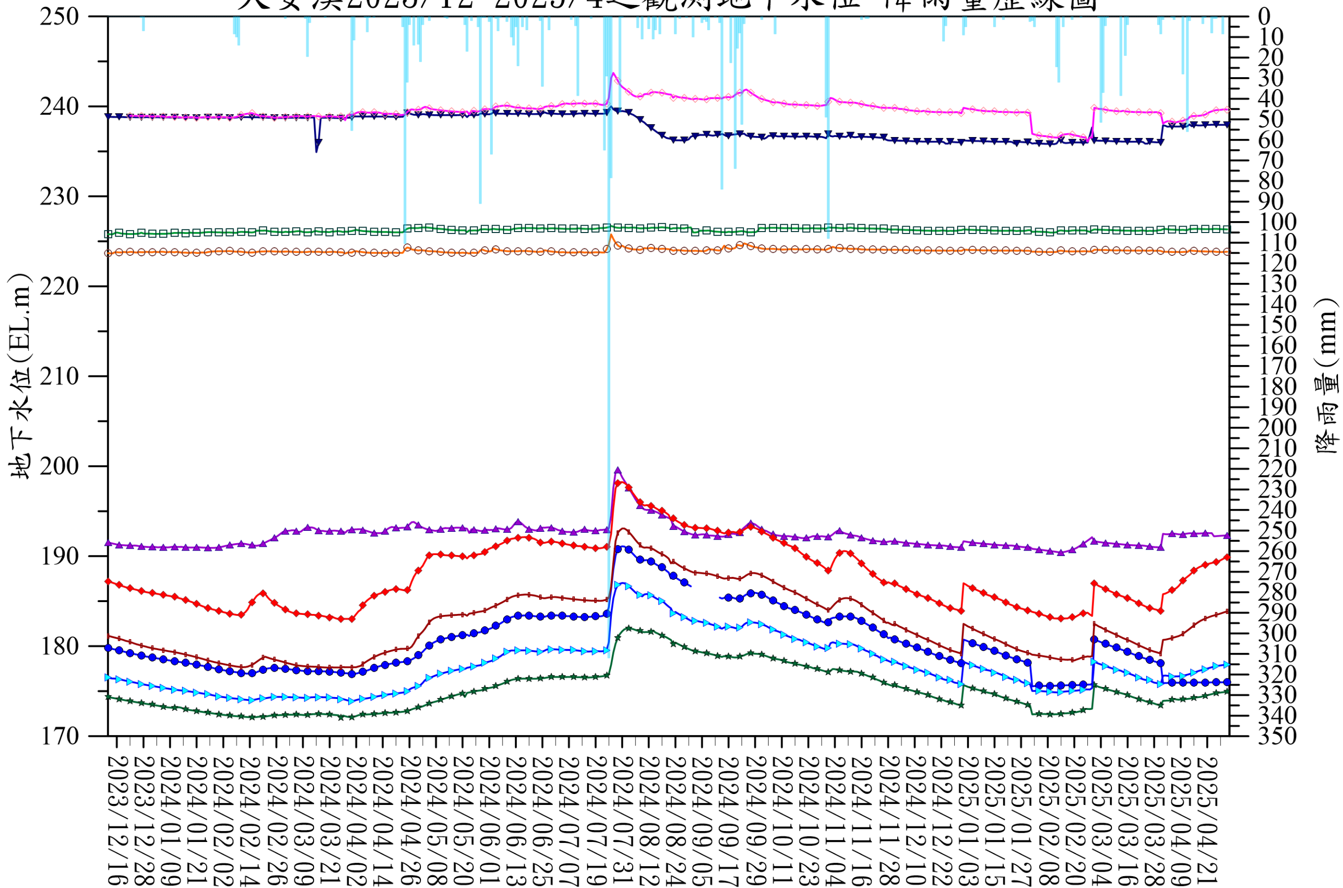
大安溪2023/12~2025/4之觀測地下水位-降雨量歷線圖
