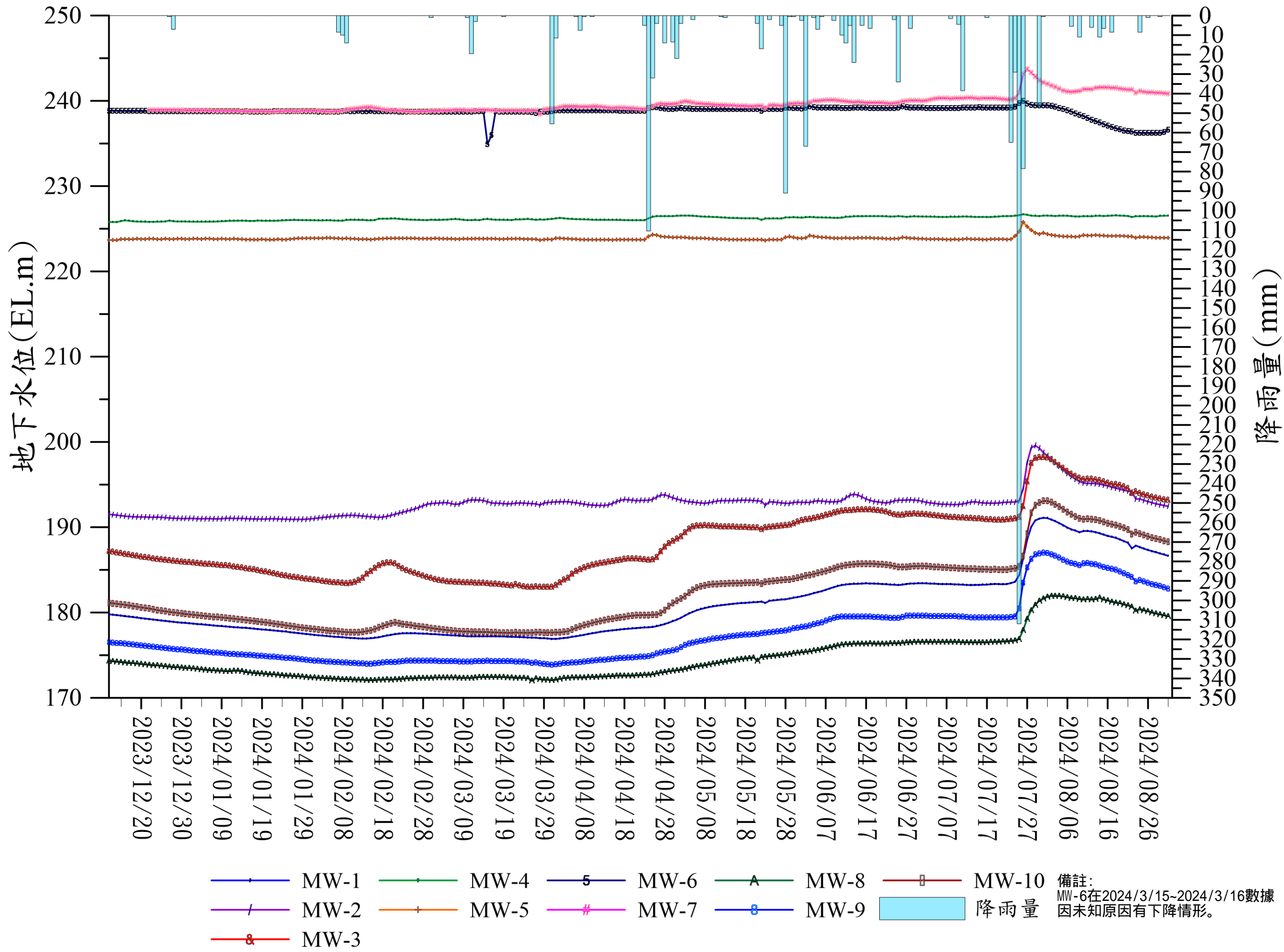
大安溪2023/12~2024/08之觀測地下水位-降雨量歷線圖
