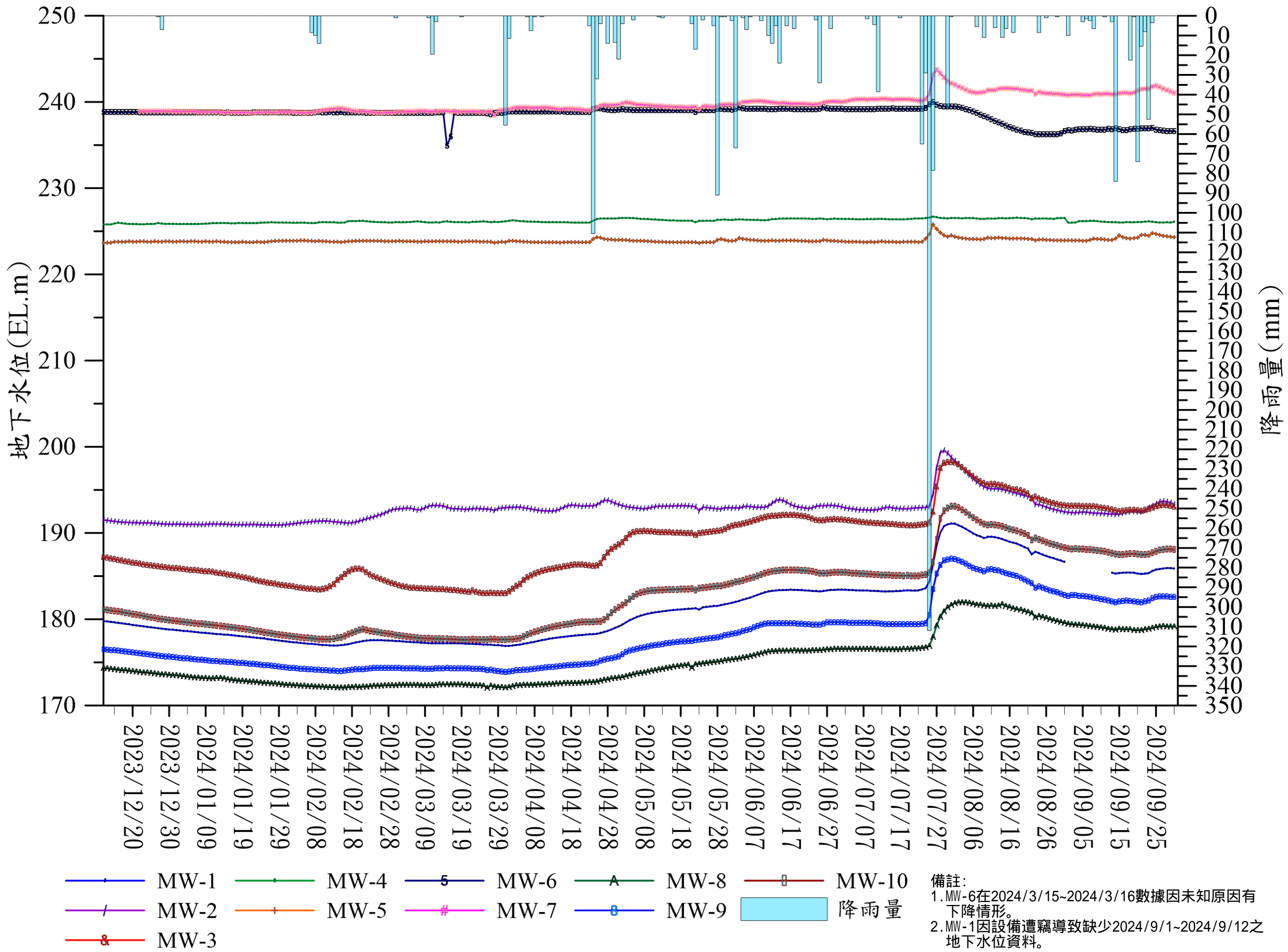
大安溪2023/12~2024/09之觀測地下水位-降雨量歷線圖
