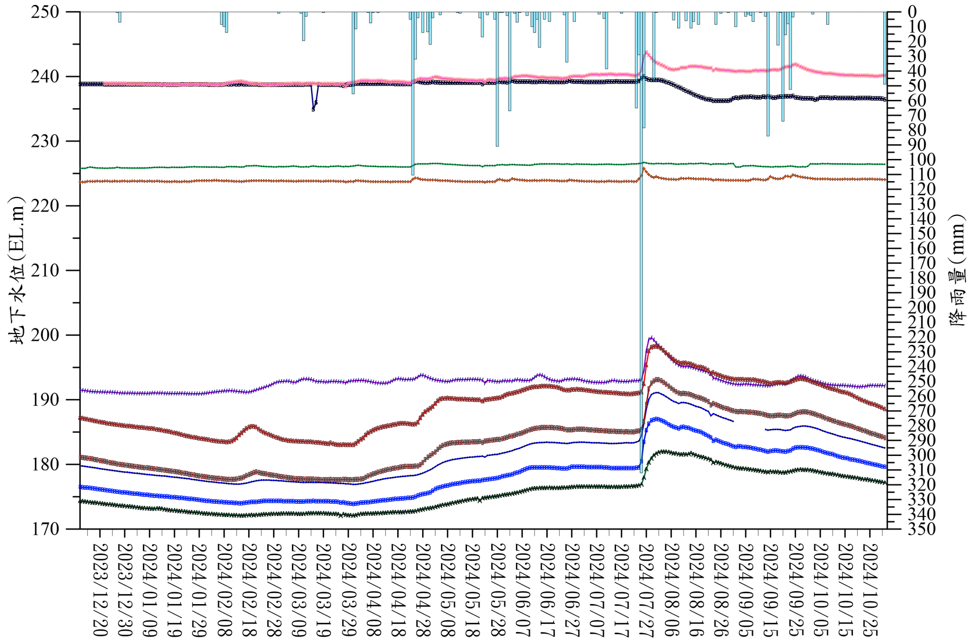
大安溪2023/12~2024/10之觀測地下水位-降雨量歷線圖
