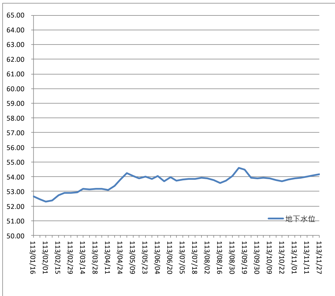
圖 4 BH-3 觀測井地下水位歷線圖
