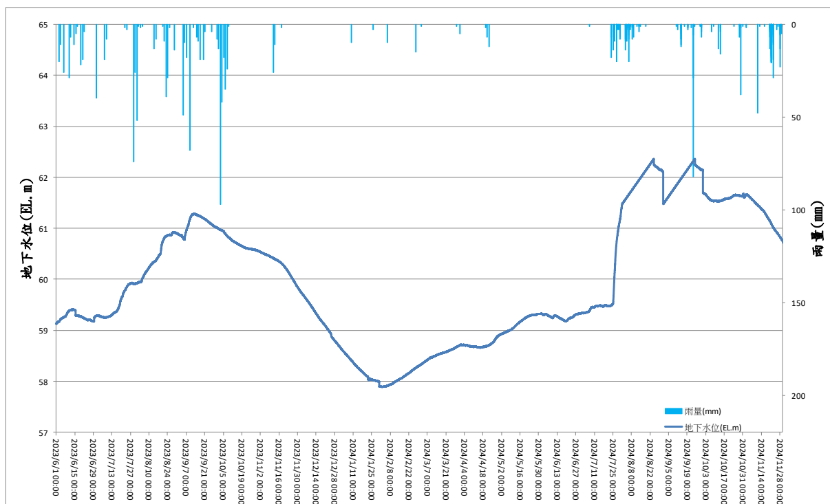
圖 11 草屯觀測井地下水位歷線圖
