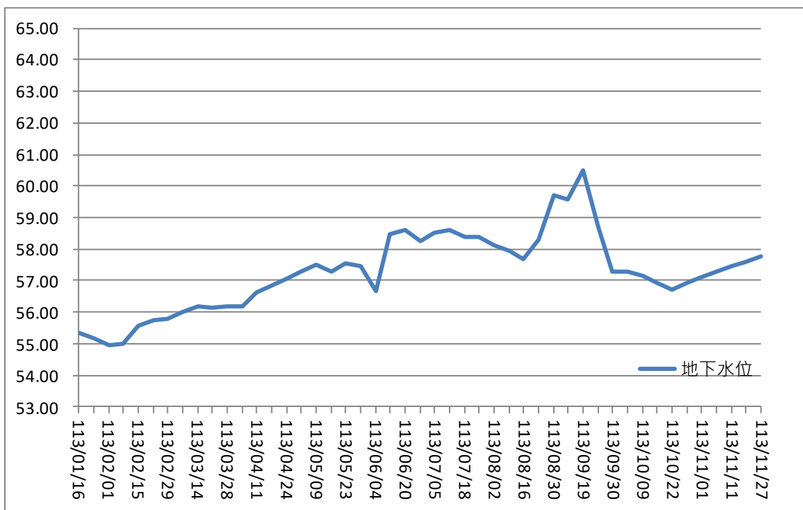
圖 2 BH-1 觀測井地下水位歷線圖
