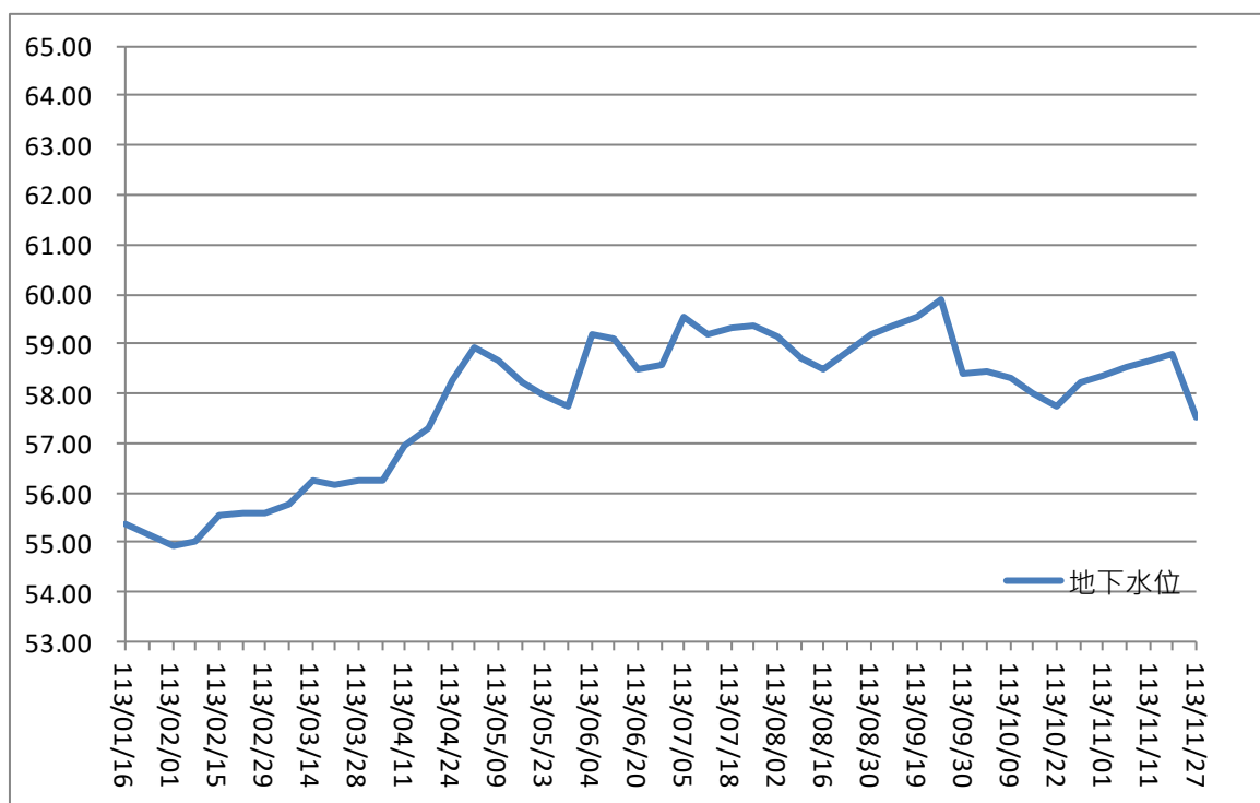
圖 3 BH-2 觀測井地下水位歷線圖
