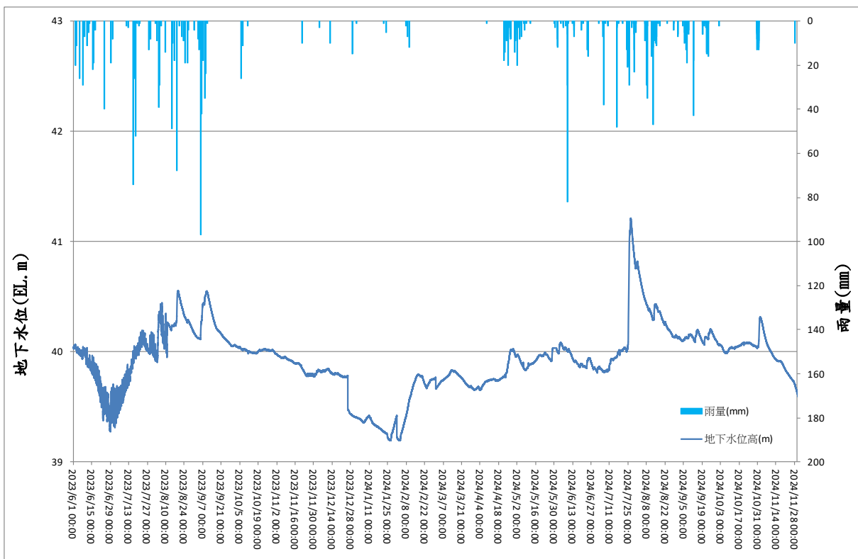
圖 8 溪岸(1)觀測井地下水位歷線圖
