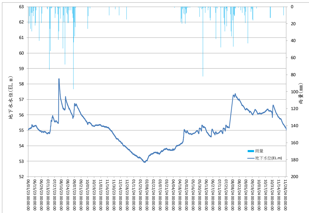
圖 7 BH-6 觀測井地下水位歷線圖
