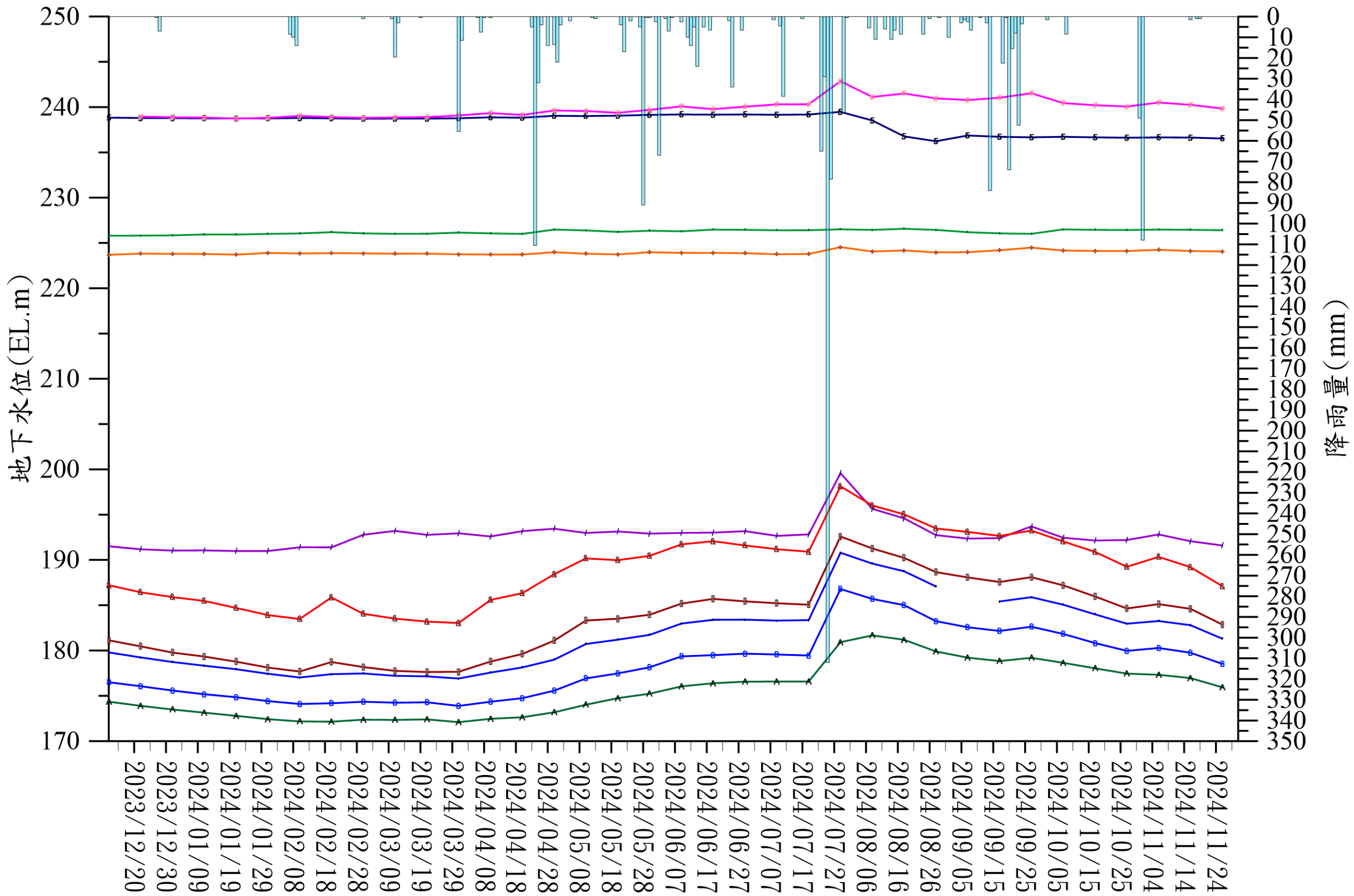
大安溪2023/12~2024/11之觀測地下水位-降雨量歷線圖
