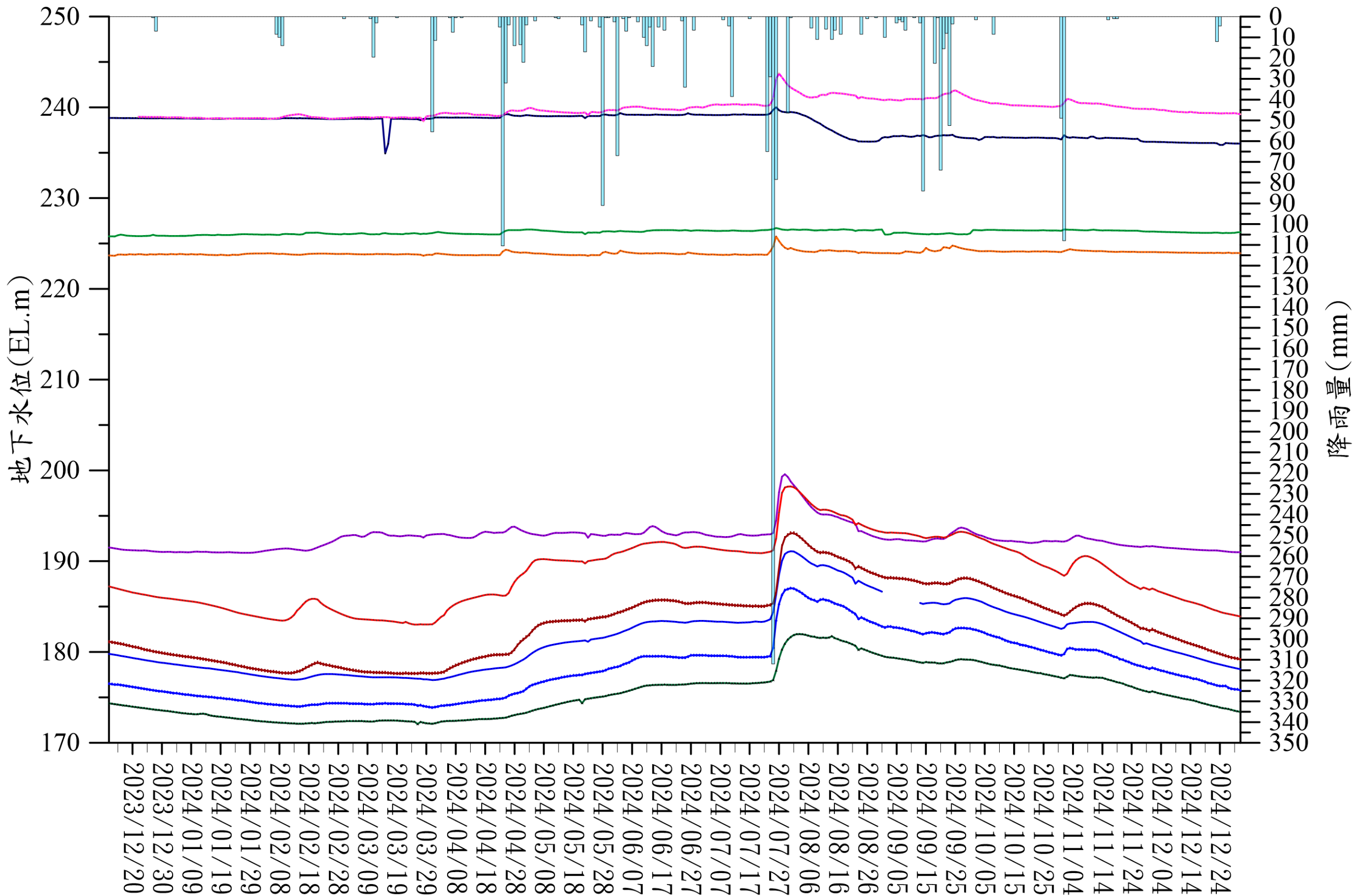
大安溪2023/12~2024/12之觀測地下水位-降雨量歷線圖
