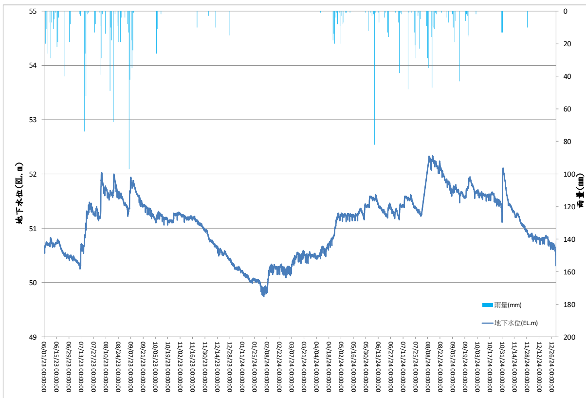
圖 5 BH-4 觀測井地下水位歷線圖
