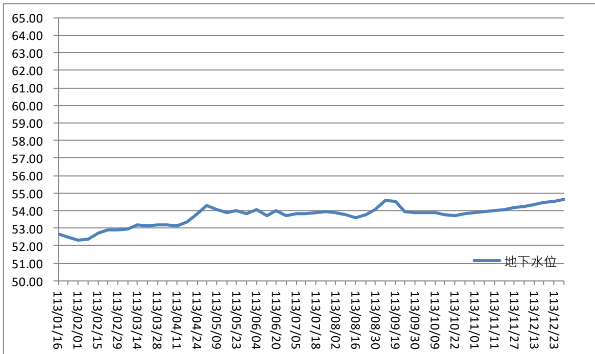
圖 4 BH-3 觀測井地下水位歷線圖
