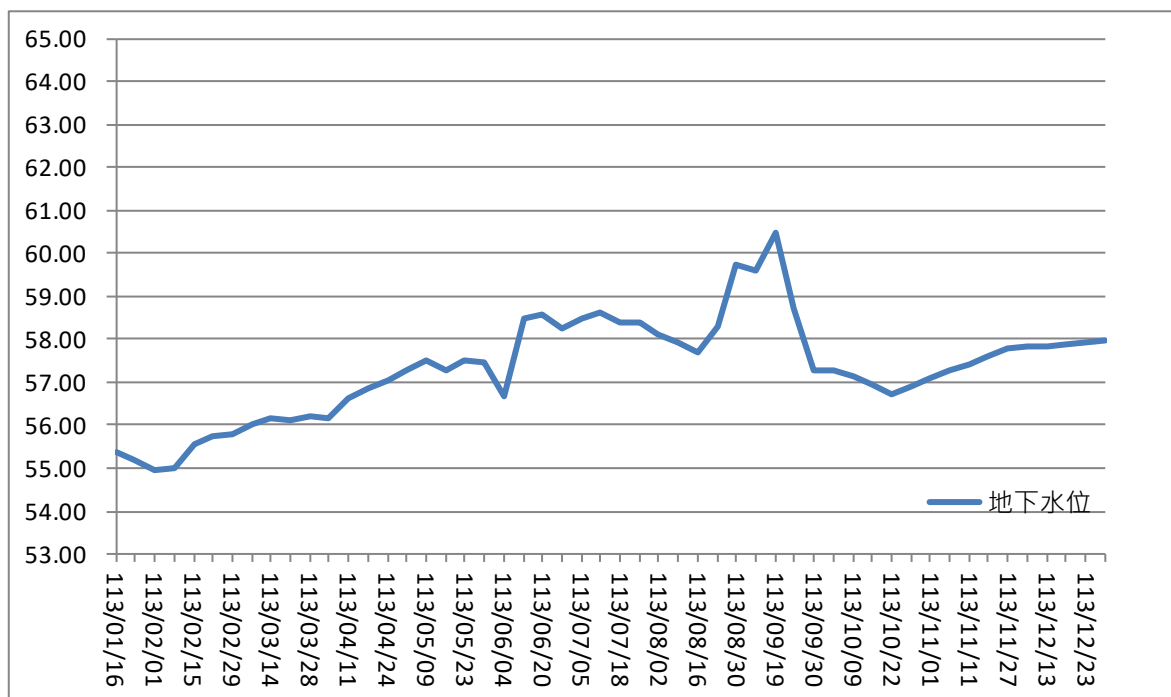
圖 2 BH-1 觀測井地下水位歷線圖
