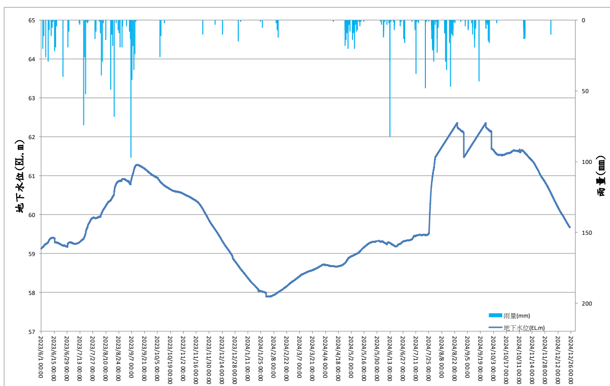
圖 11 草屯觀測井地下水位歷線圖
