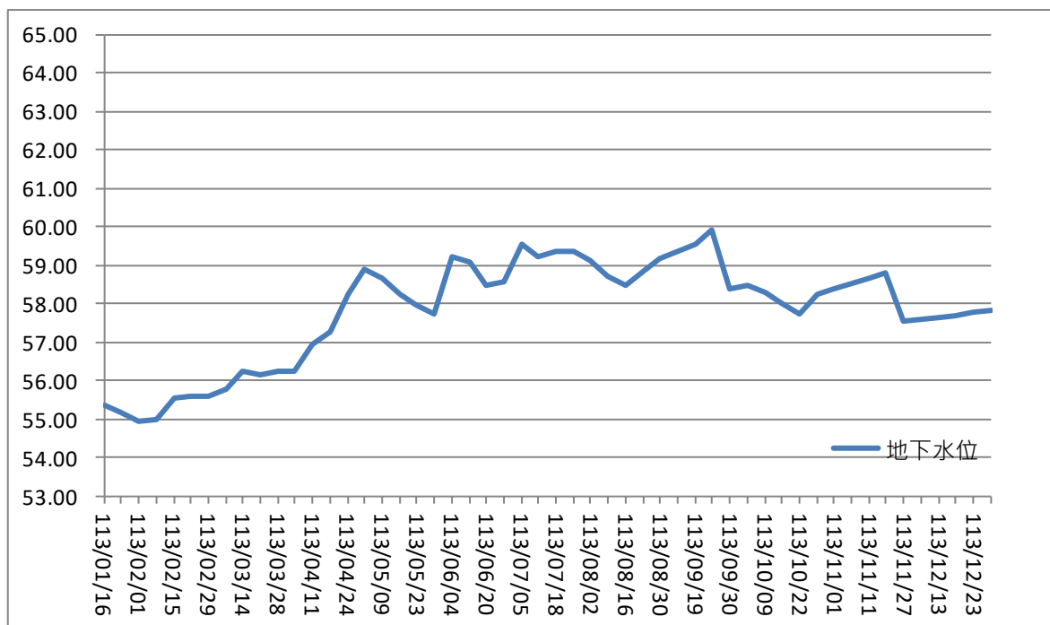
圖 3 BH-2 觀測井地下水位歷線圖
