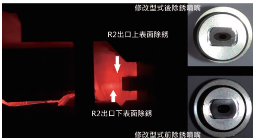
圖 4、粗軋區除銹噴嘴型式修正減少噴水量
