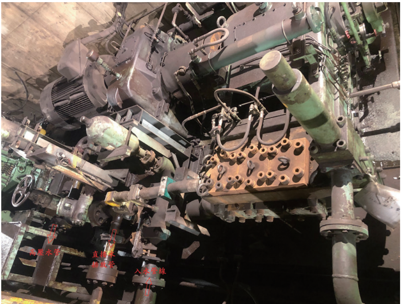
圖 3、除銹水系統節水設備
