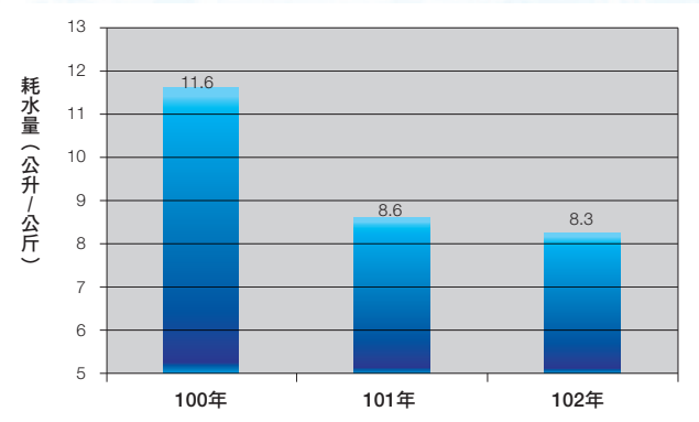
近三年滾筒式省水標章洗衣機平均耗水量圖
